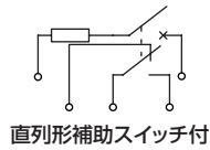
直列形補助スイッチ付
