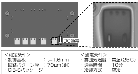
図4. 制御基板パターンの発熱評価方法
