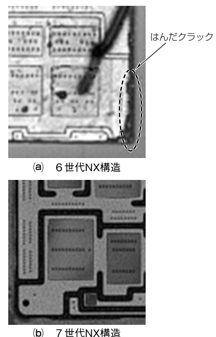
図3. サーマルサイクル後のSAT画像
