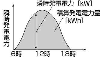
●1日の瞬時発電電力の推移 (一例)
