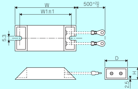
FR-ABR-0.4K~7.5K、H0.4K~H7.5K
