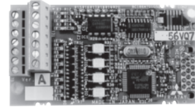
700シリーズ内蔵オプション例:FR-A7AY
