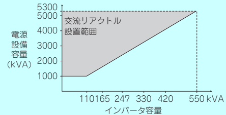
<大容量電源トランス使用時のリアクトルの選定>
