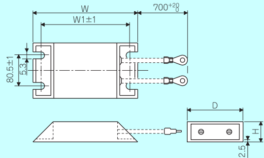
FR-ABR-11K~22K、H11K~H22K
