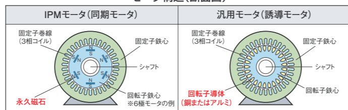
モータ構造(断面図)
