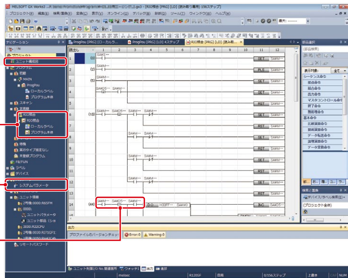
GX Works3上で安全制御用のプログラムファイルを管理
