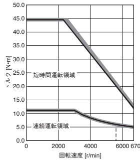
HK-ST3534W トルクアップ
