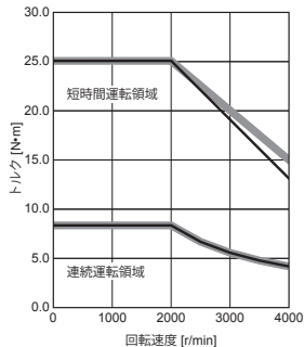
HK-ST172W (注2) 標準トルク
