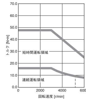
HK-ST503W 標準トルク
