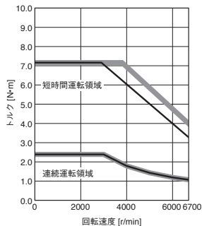
HK-MT7M3W 標準トルク
