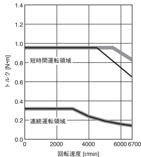
HK-MT13W 標準トルク
