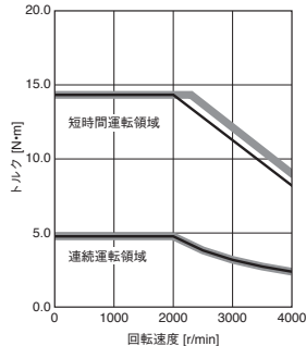
HK-ST102W (注2) 標準トルク
