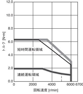
HK-KT63UW 標準トルク
