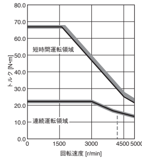
HK-RT7034W 標準トルク
