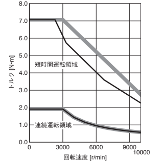
HK-MT63VW トルクアップ
