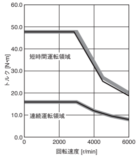
HK-RT5034W 標準トルク
