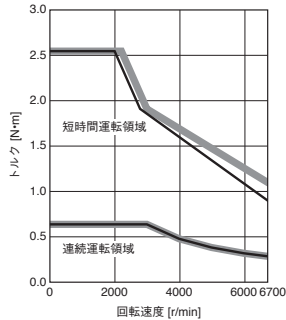
HK-KT23UW トルクアップ
