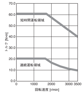
HK-ST352W トルクアップ
