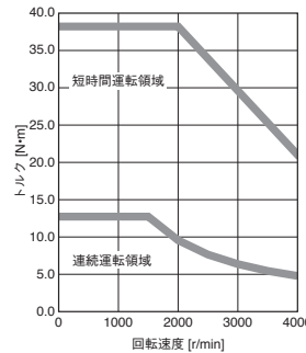
HK-ST202W トルクアップ
