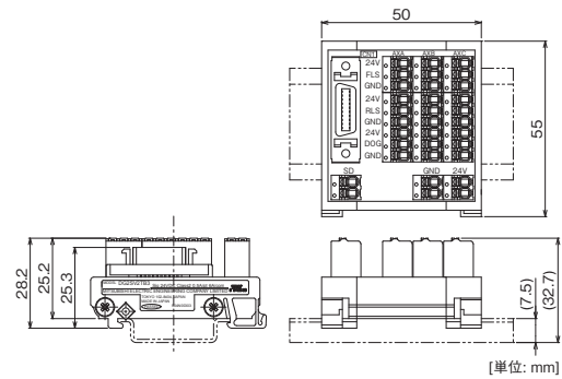
■ DG2SV2TB3 (3軸サーボアンプ用)
