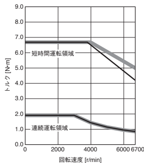
HK-KT63W 標準トルク
