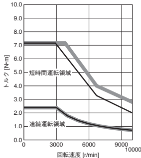
HK-MT7M3VW 標準トルク
