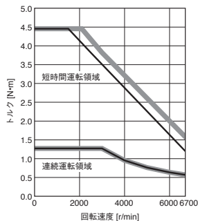
HK-MT43W トルクアップ
