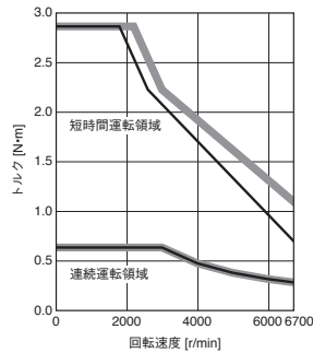
HK-KT23W トルクアップ
