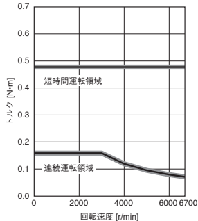
HK-MT053W 標準トルク
