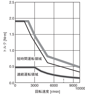
HK-MT1M3VW トルクアップ
