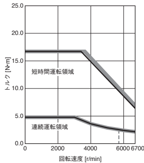
HK-KT1534W 標準トルク
