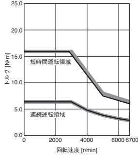
HK-RT2034W 標準トルク
