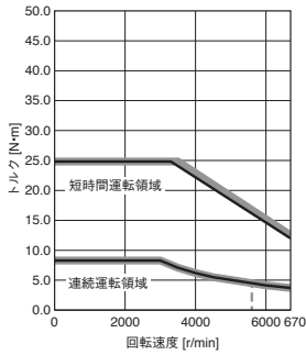
HK-ST3534W 標準トルク
