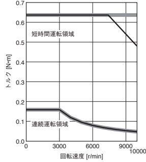
HK-MT053VW トルクアップ
