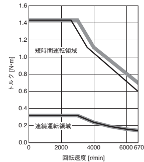
HK-KT13UW トルクアップ
