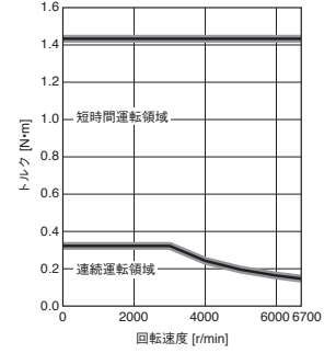
HK-KT13W トルクアップ
