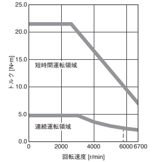
HK-KT153W トルクアップ
