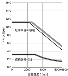
HK-KT103W (注2) 標準トルク
