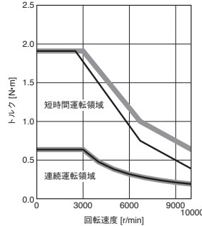
HK-MT23VW 標準トルク
