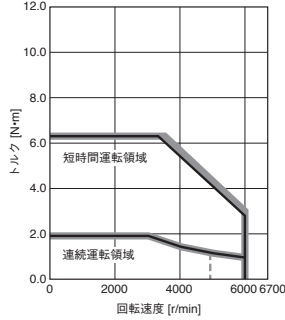
HK-KT634UW 標準トルク
