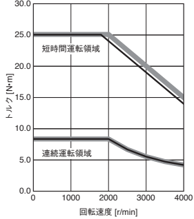
HK-ST1724W 標準トルク
