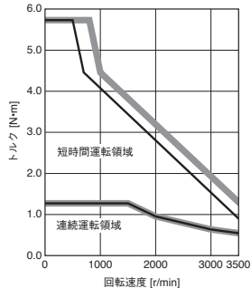
HK-KT434W トルクアップ
