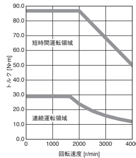
HK-ST502W トルクアップ
