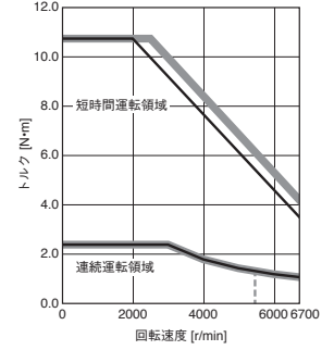
HK-KT7M3UW トルクアップ
