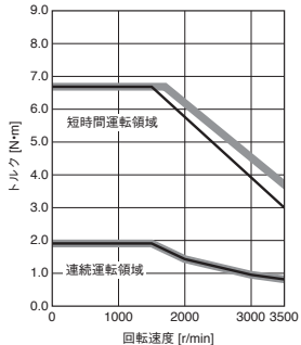
HK-KT634W 標準トルク
