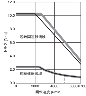
HK-KT63UW トルクアップ
