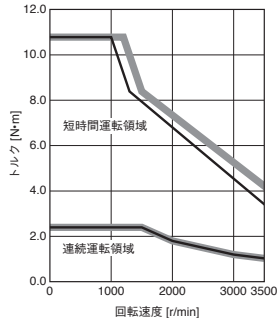
HK-KT7M34W トルクアップ
