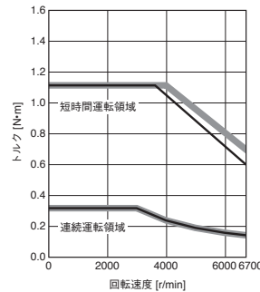
HK-KT13UW 標準トルク
