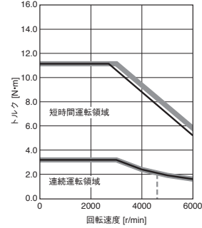
HK-KT1034UW 標準トルク
