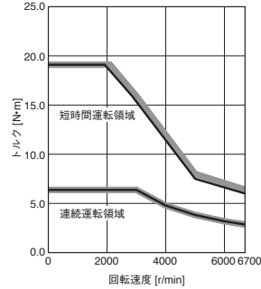
HK-RT2034W トルクアップ
