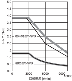
HK-MT43VW 標準トルク
