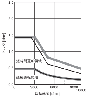
HK-MT1M3VW 標準トルク
