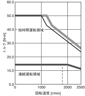
HK-ST3024W トルクアップ
