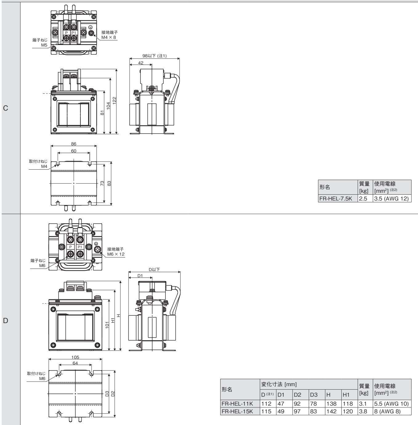
外形寸法図
