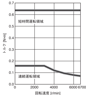
HK-MT053W トルクアップ
