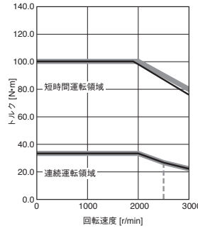
HK-ST7024W 標準トルク
