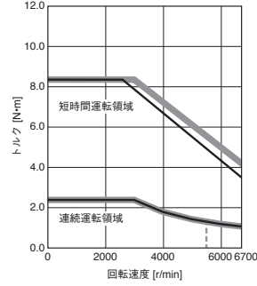
HK-KT7M3UW 標準トルク
