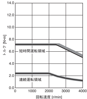
HK-ST52W 標準トルク
