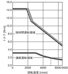
HK-KT1034W トルクアップ
