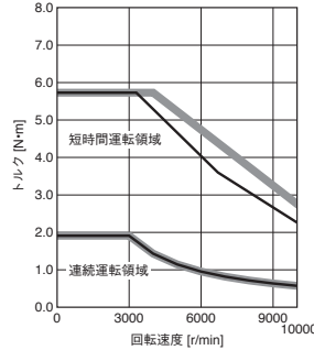
HK-MT63VW 標準トルク
