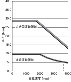
HK-ST2024W 標準トルク
