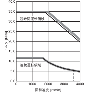
HK-ST2024AW トルクアップ
