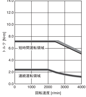
HK-ST524W 標準トルク
