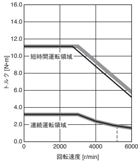
HK-KT103UW (注2) 標準トルク
