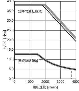
HK-ST2024W トルクアップ
