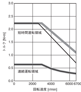
HK-KT23W 標準トルク
