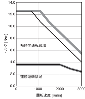
HK-ST7M2UW トルクアップ
