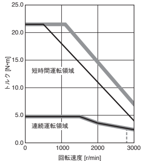
HK-KT1534W トルクアップ
