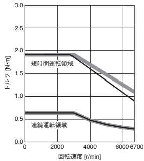
HK-KT23UW 標準トルク
