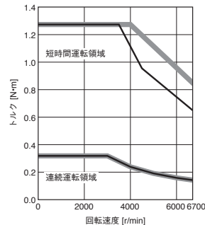
HK-MT13W トルクアップ
