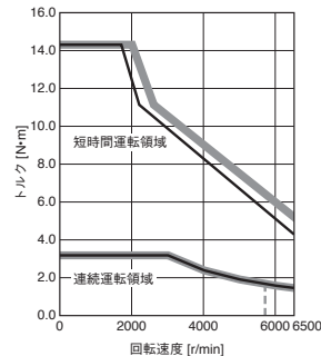
HK-KT103W (注2) トルクアップ
