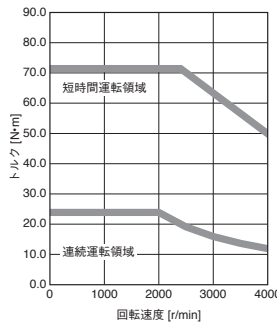
HK-ST502W 標準トルク
