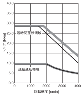
HK-ST202W (注2) 標準トルク
