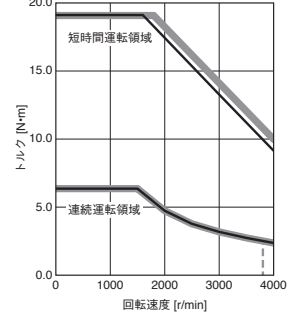
HK-ST1024W トルクアップ
