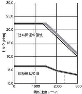
HK-KT2034W (注2) 標準トルク
