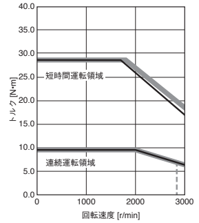
HK-KT202W (注2) 標準トルク
