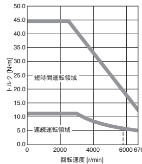
HK-ST353W トルクアップ
