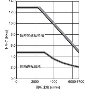
HK-RT1534W トルクアップ
