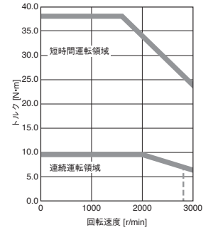
HK-KT202W トルクアップ
