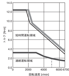
HK-MT103W (注2) トルクアップ
