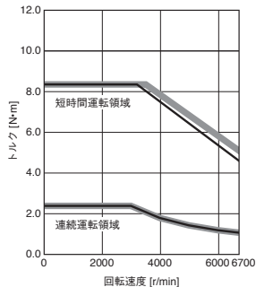
HK-KT7M3W 標準トルク
