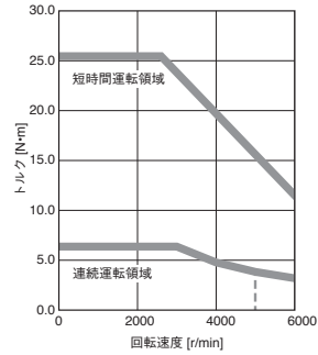
HK-KT203W トルクアップ
