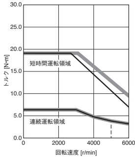
HK-KT203W (注2) 標準トルク
