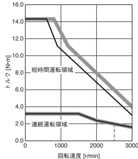
HK-KT1034W トルクアップ
