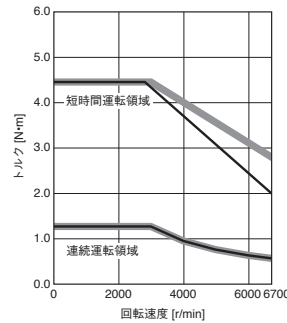
HK-KT43W 標準トルク
