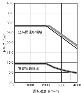
HK-ST202AW (注2) 標準トルク
