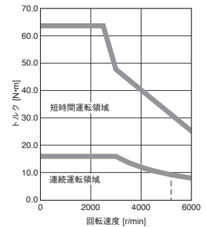
HK-ST503W トルクアップ
