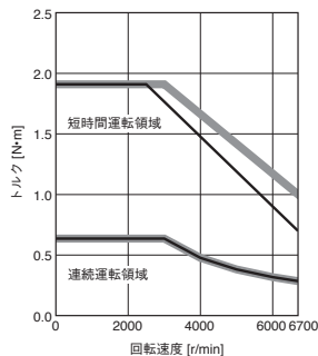
HK-MT23W 標準トルク
