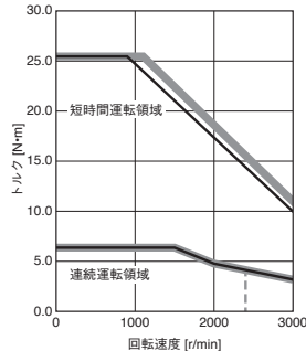
HK-KT2034W (注2) トルクアップ
