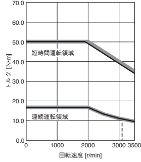
HK-ST3524W 標準トルク
