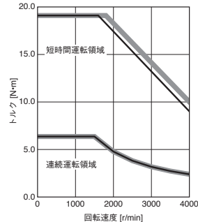
HK-ST102W (注2) トルクアップ
