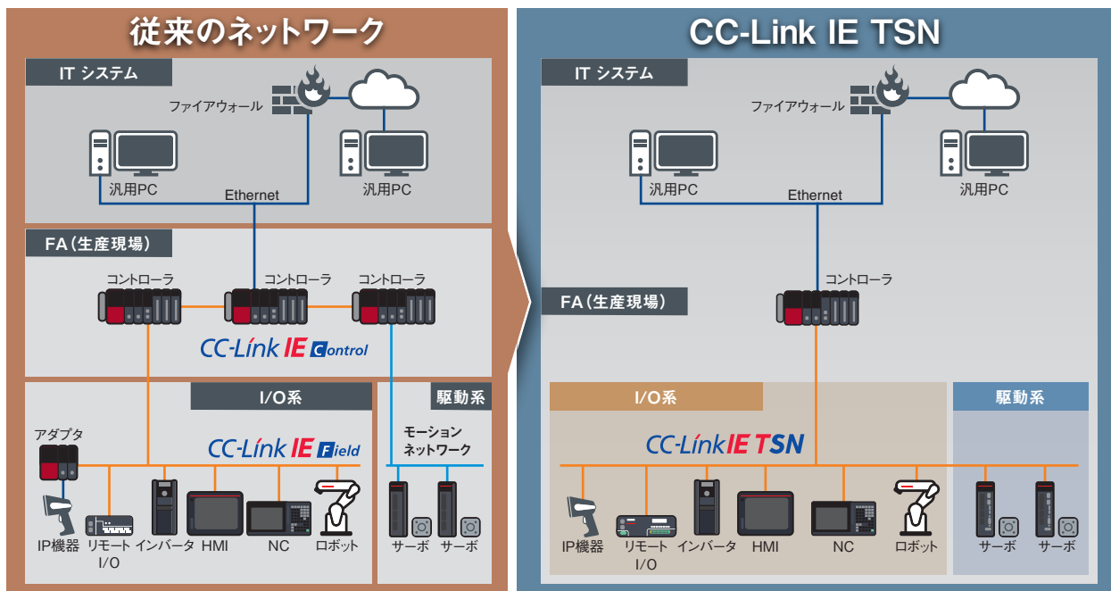
ネットワーク全体構成イメージ (将来対応の機能、製品を含む)
