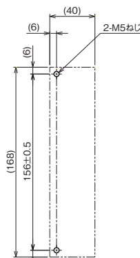
取付け穴加工図
