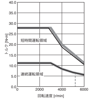
HK-RT3534W 標準トルク
