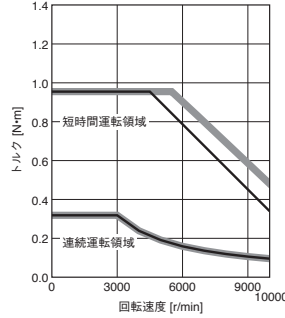
HK-MT13VW 標準トルク
