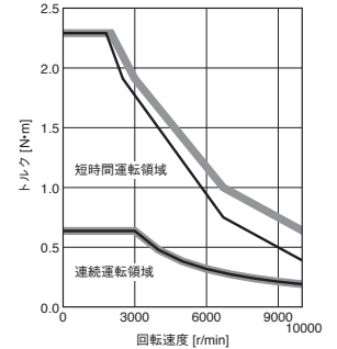
HK-MT23VW トルクアップ
