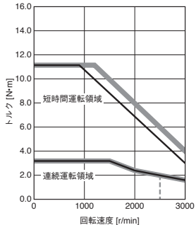
HK-KT1034W 標準トルク
