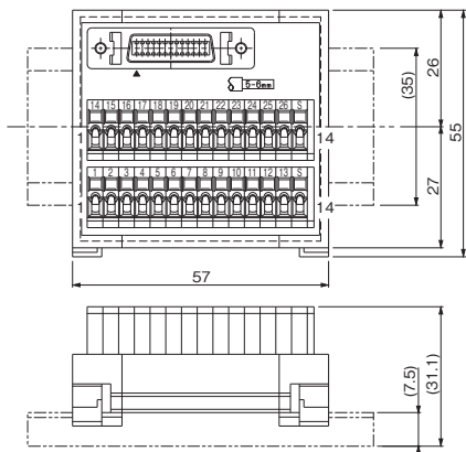
外形寸法図 (注1) [単位: mm]
