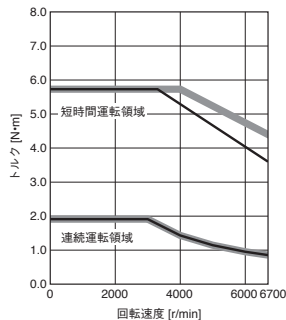
HK-MT63W 標準トルク
