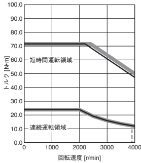
HK-ST5024W 標準トルク
