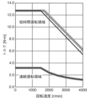
HK-ST52W トルクアップ
