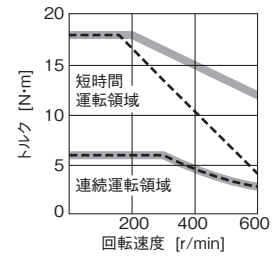
TM-RG2M004E30, TM-RU2M004E30 (注1, 2, 3, 4) (トルク増大時)
