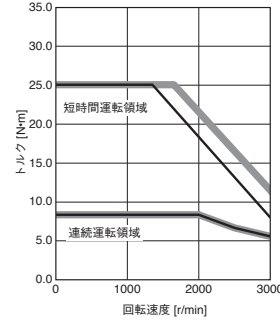
HK-ST172UW (注2) 標準トルク
