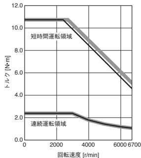
HK-KT7M3W トルクアップ
