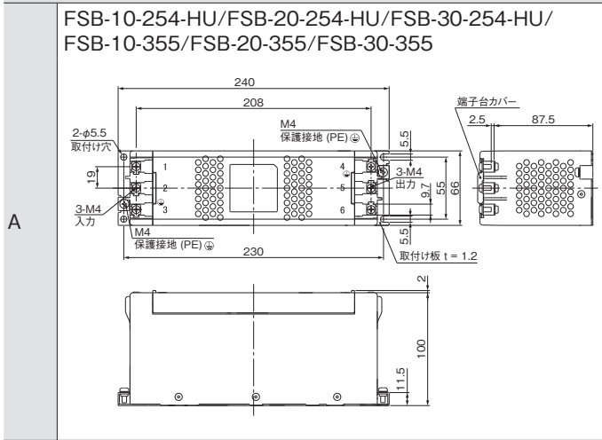
外形寸法図
