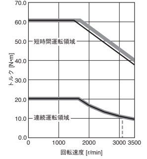
HK-ST3524W トルクアップ
