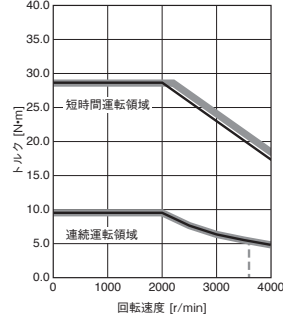
HK-ST2024AW 標準トルク
