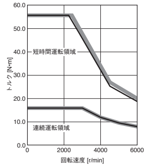
HK-RT5034W トルクアップ
