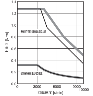
HK-MT13VW トルクアップ
