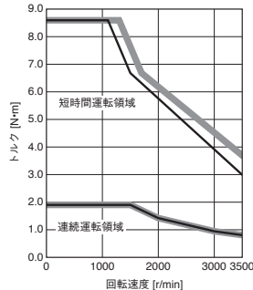
HK-KT634W トルクアップ
