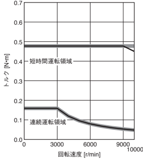
HK-MT053VW 標準トルク
