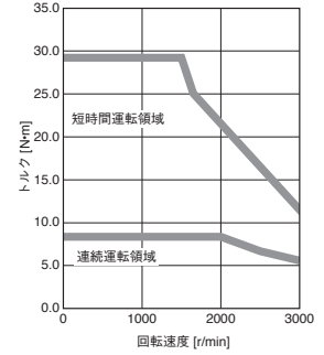
HK-ST172UW トルクアップ
