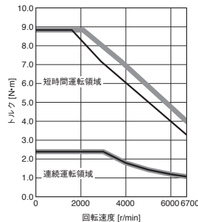
HK-MT7M3W トルクアップ
