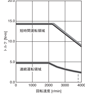
HK-ST1024W 標準トルク
