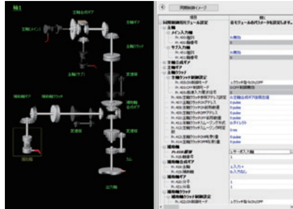
アドバンス同期制御用データ (イメージ図)
