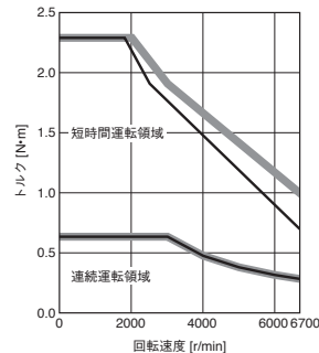
HK-MT23W トルクアップ
