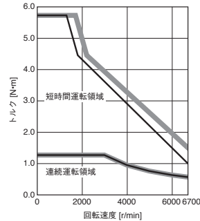
HK-KT43UW トルクアップ
