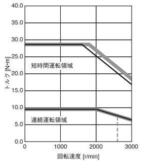
HK-KT2024W 標準トルク
