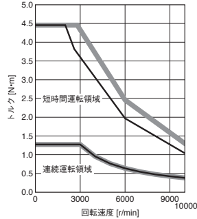
HK-MT43VW トルクアップ
