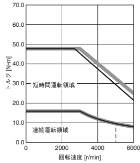
HK-ST5034W 標準トルク
