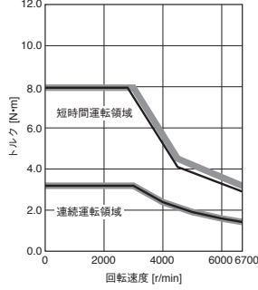
HK-RT1034W 標準トルク
