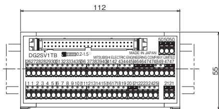
外形寸法図 [単位: mm]
