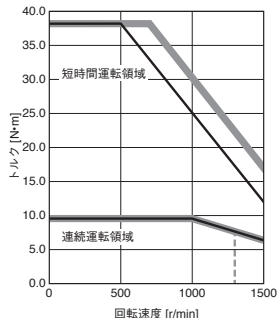
HK-KT2024W (注2) 標準トルク
