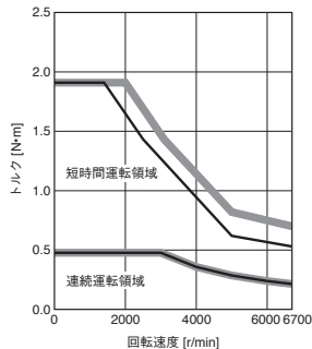
HK-MT1M3W トルクアップ
