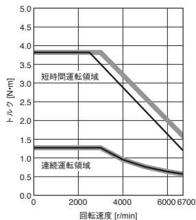
HK-MT43W 標準トルク
