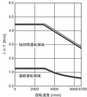
HK-KT434W 標準トルク
