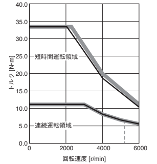
HK-RT3534W トルクアップ
