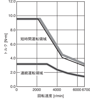
HK-RT1034W トルクアップ
