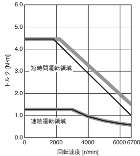
HK-KT43UW 標準トルク
