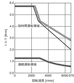
HK-KT43W トルクアップ
