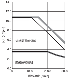
HK-ST7M2UW 標準トルク
