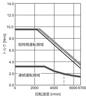
HK-MT103W (注2) 標準トルク
