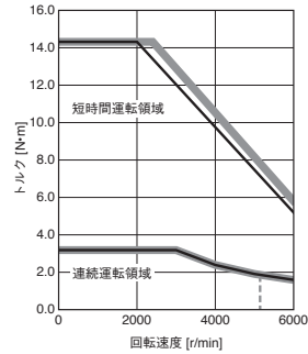
HK-KT103UW (注2) トルクアップ
