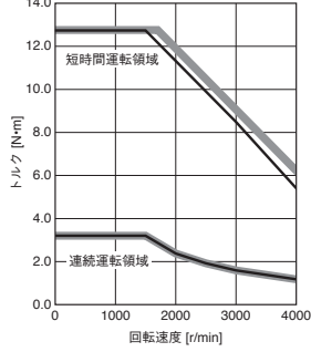
HK-ST524W トルクアップ
