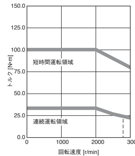
HK-ST702W 標準トルク
