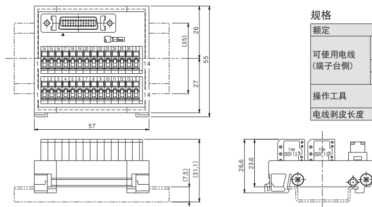
外形尺寸图 (注1)
