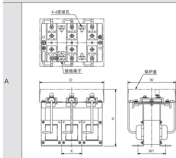
外形尺寸图
