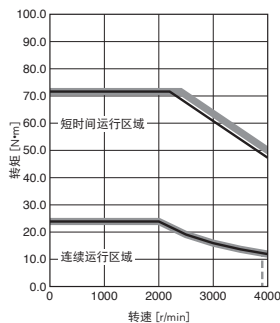
HK-ST5024WJ 标准转矩
