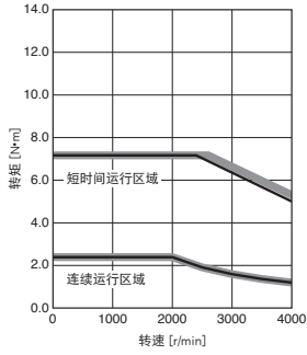
HK-ST52WJ 标准转矩
