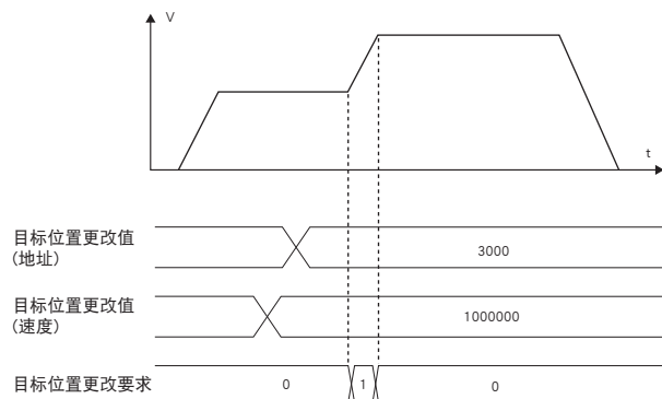
[时间图]
