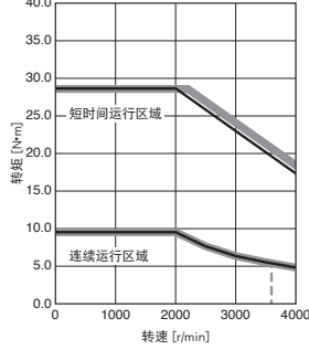
HK-ST2024AWJ 标准转矩
