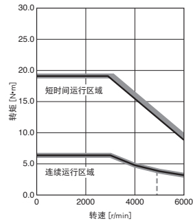
HK-KT2034WJ 标准转矩
