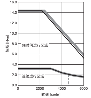
HK-KT1034UWJ 转矩提升
