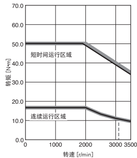
HK-ST3524WJ 标准转矩
