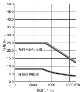
HK-ST3534WJ 标准转矩
