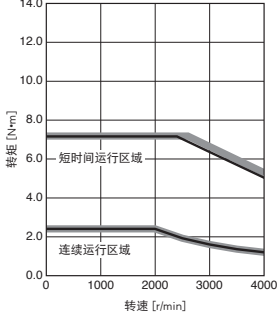
HK-ST524WJ 标准转矩
