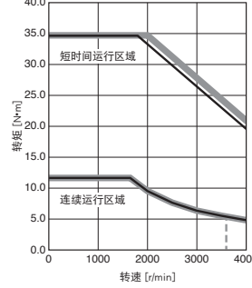
HK-ST2024AWJ 转矩提升
