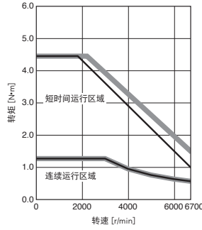
HK-KT43UWJ 标准转矩
