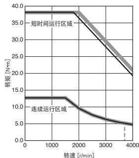
HK-ST2024WJ 转矩提升
