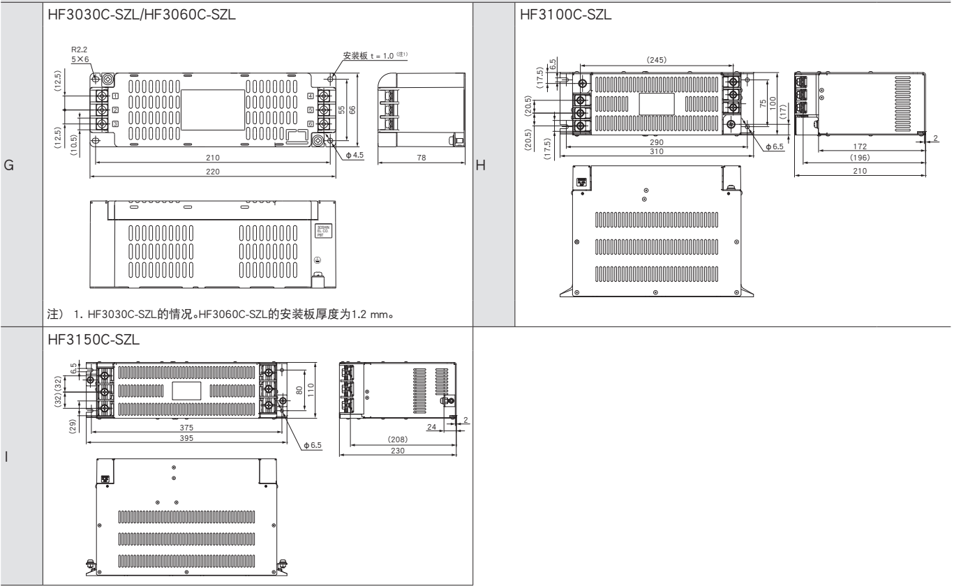
外形尺寸图
