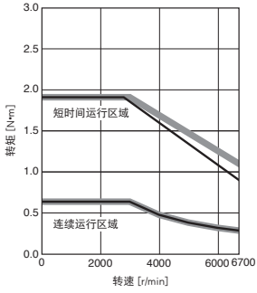
HK-KT23UWJ 标准转矩
