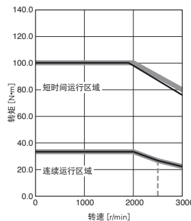
HK-ST7024WJ 标准转矩
