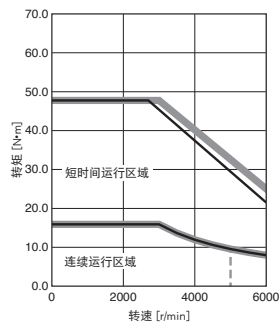
HK-ST5034WJ 标准转矩
