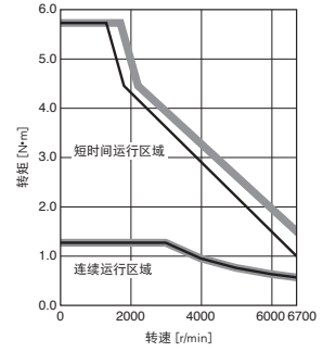
HK-KT43UWJ 转矩提升
