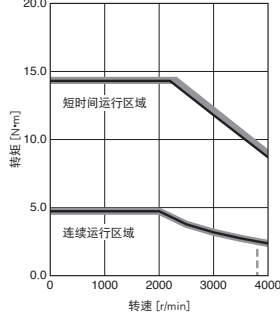
HK-ST1024WJ 标准转矩
