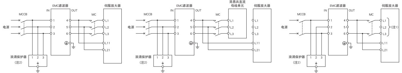
连接图
