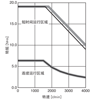
HK-ST102WJ (注2) 转矩提升
