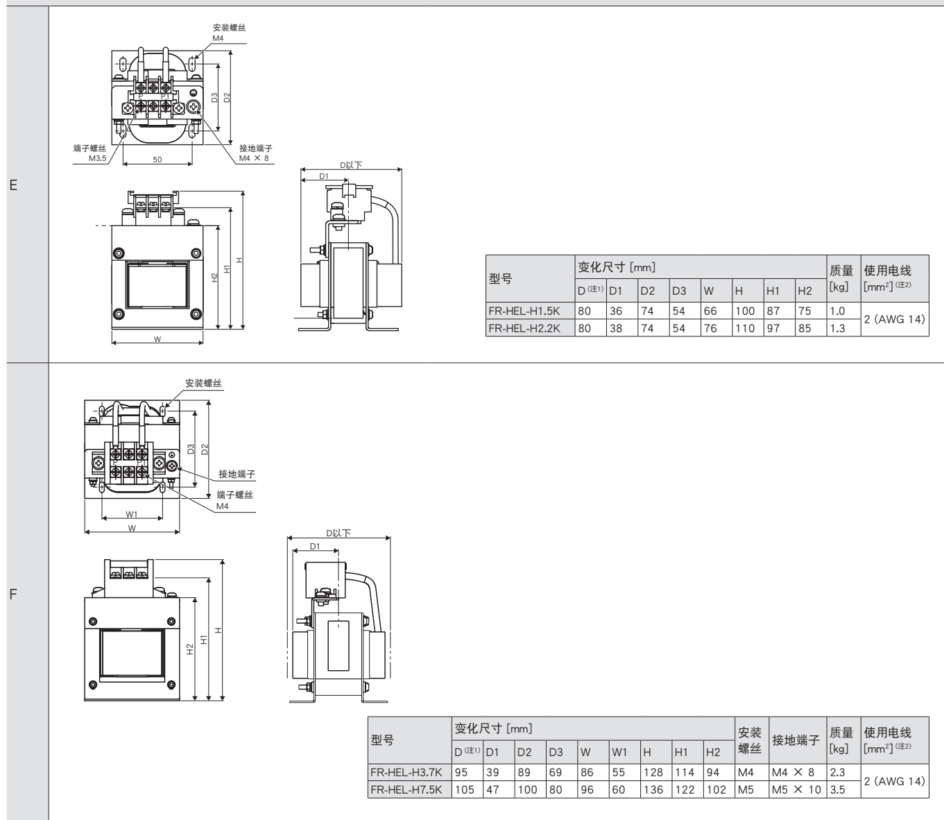
外形尺寸图
