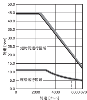
HK-ST3534WJ 转矩提升
