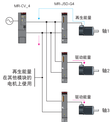
[直流共母线连接]
