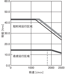
HK-ST3024WJ 标准转矩
