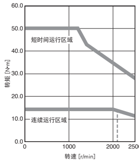
HK-ST302WJ 转矩提升
