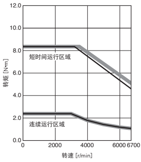
HK-KT7M3WJ 标准转矩
