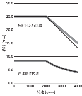
HK-ST172WJ (注2) 标准转矩
