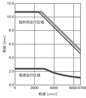
HK-KT7M3WJ 转矩提升
