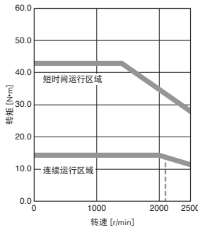
HK-ST302WJ 标准转矩
