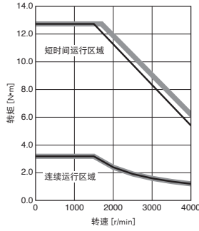
HK-ST52WJ 转矩提升
