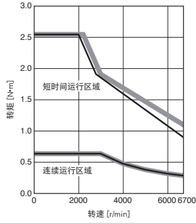
HK-KT23UWJ 转矩提升
