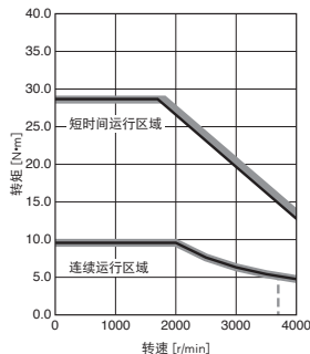
HK-ST2024WJ 标准转矩
