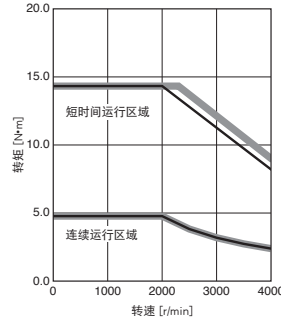
HK-ST102WJ (注2) 标准转矩
