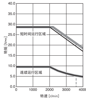
HK-ST202AWJ (注2) 标准转矩
