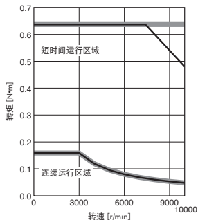
HK-MT053VWJ 转矩提升
