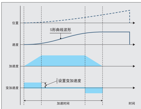
变加速度加减速方式
