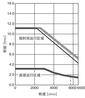
HK-KT103WJ (注2) 标准转矩
