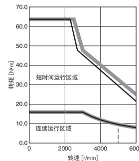
HK-ST5034WJ 转矩提升
