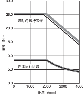
HK-ST1724WJ 标准转矩
