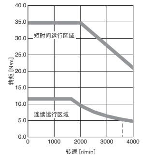
HK-ST202AWJ 转矩提升
