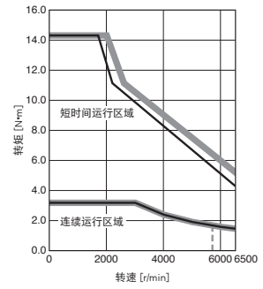
HK-KT103WJ (注2) 转矩提升
