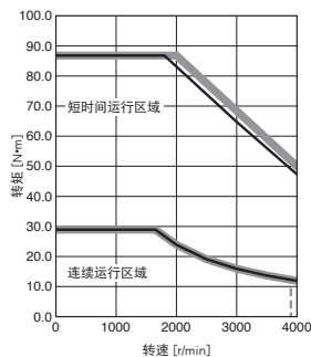
HK-ST5024WJ 转矩提升
