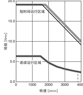
HK-ST1024WJ 转矩提升
