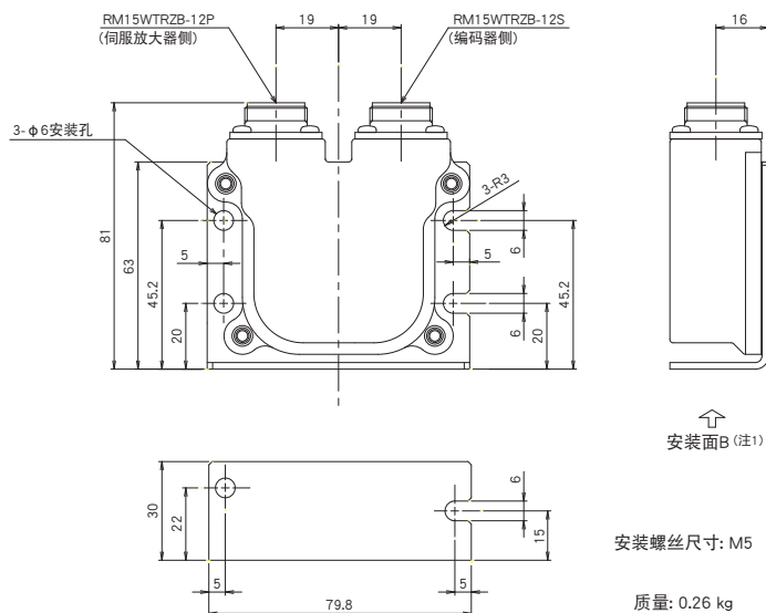
外形尺寸图 [单位: mm]
