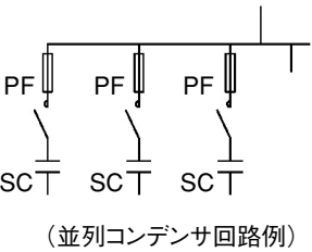
（並列コンデンサ回路例）
