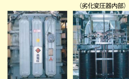
(劣化変圧器内部)
