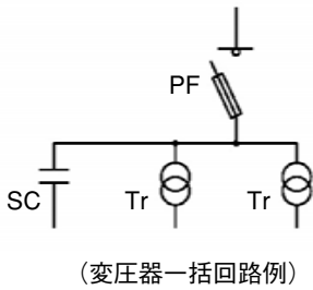
（変圧器一括回路例）
