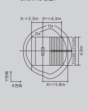
図1 器具配置と照度範囲 (表1の器具を高さ2.5mに取付けた場合)
