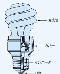
D形の構造図（スパイラルピカファン D15形）
