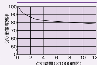
コンパクト形蛍光ランプの 光束維持特性（FPL36□）
