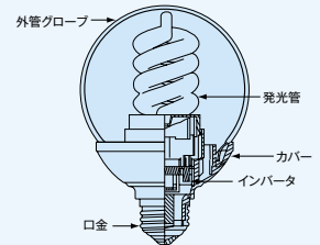
D形の構造図（スパイラルピカファン D15形）
