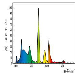
スーパークリア色 (EDX) Ra84
