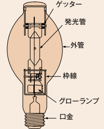
高圧ナトリウムランプの構造図
