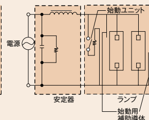
(d) 始動器内蔵高圧ナトリウムランプ (ハイルックス-W・L) (始動器:バイメタルスイッチ+ヒーター)
