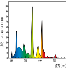
3波長形昼白色
