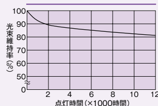
Hf32Wランプ（ルビカラインブラチナ） の光束維持特性（FHF32□-H3）
