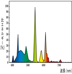
スーパークリア色 (EDX) Ra84
