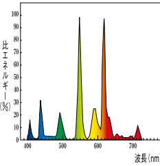
3波長形電球色 (EX-L) Ra84
