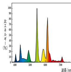
昼白色 (EDL) Ra99
