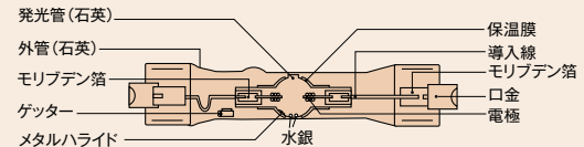
HQIランプの構造図 (両口金タイプ)
