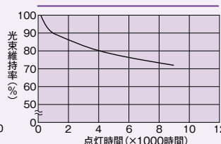
コンパクト形蛍光ランプの 光束維持特性（FPL36□）
