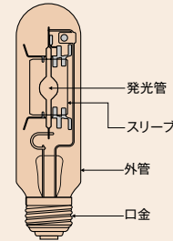
水銀ランプの構造図
