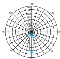
LEL100V5W/CW/RF (昼光色)
