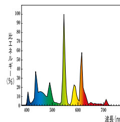
3波長形昼白色 (EX-N, EN) Ra84
