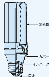
D形の構造図（ルピカボールE D15形）
