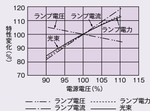
図1 電源電圧変動による 光束・特性変化例(FL40S)
