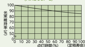
図6 ハイルックス・L (NH360F・L)
