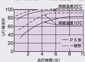
光束立ち上がり特性(直管40形)
