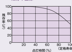
残存率曲線
