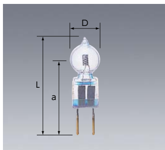
□金:GY6.35 単位:mm
