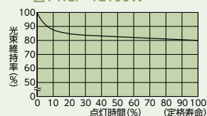
図3 HQI®ランプ (HQI-TS 150W/NDL)
