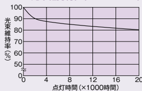
Hf32Wランプ(ルビカラインプラチナ) の光束維持特性 (FHF32□-H3)
