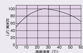
周囲温度による光束変化 (FHF)
