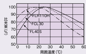
周囲温度による光束変化
