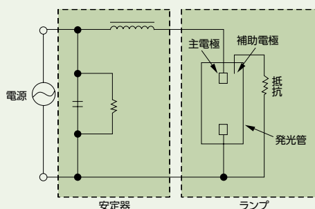
水銀ランプの始動機構
