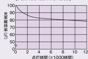
40Wランプの光束維持特性 [FLR40S・□/M( /36)]
