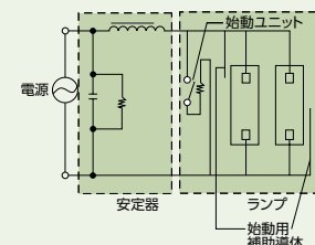
(d)始動器内蔵形高圧ナトリウムランプ (ハイルックス・W・L) (始動器:バイメタルスイッチ+ヒーター)
