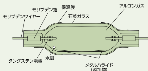
メタルハライドランプの発光管
