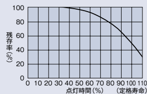
残存率曲線
