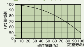
図10 高圧ナトリウムランプ・水銀ランプ
