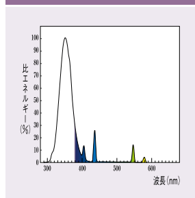
分光分布
