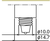
□金:EZ10 単位:mm
