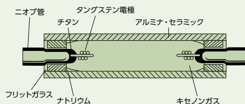
高圧ナトリウムランプの発光管
