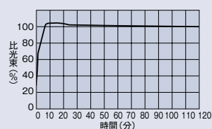
スパイラルピカミニの光束立ち上がり特性(A15形、周囲温度25℃)
