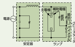
(d)始動器内蔵形高圧ナトリウムランプ (ハイルックス・W・L) (始動器:バイメタルスイッチ+ヒーター)
