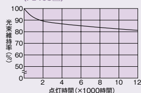
40Wランプの光束維持特性 (FL40S□)
