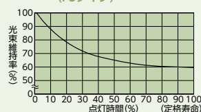
図5 マルチスター・L2 (PSタイプ)
