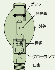
高圧ナトリウムランプの構造図
