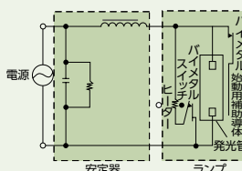
(c)始動器内蔵形高圧ナトリウムランプ (ハイルックスL・ハイルックスDL) (始動器:バイメタルスイッチ+ヒーター)
