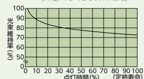
図4 マルチスター・L2 (MF400・L-J2/BU-P)
