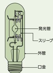
水銀ランプの構造図
