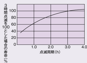
ランプの点滅周期と寿命
