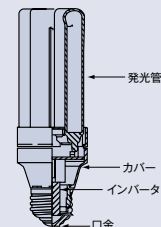
D形の構造図 (ルピカボールE D15形)
