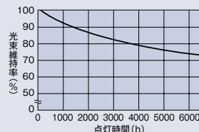
光束維持特性
