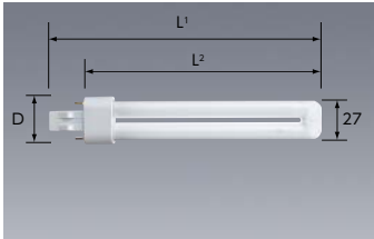
(上記写真は13Wタイプで口金はGX23です。)
