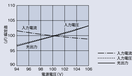
電源電圧変動特性
