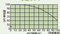
図8 高圧ナトリウムランプ・水銀ランプ
