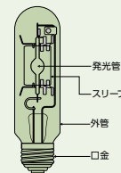
水銀ランプの構造図
