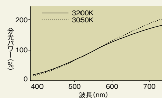
分光分布
