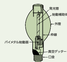
高圧ナトリウムランプの構造図
