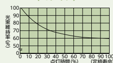
図5 水銀ランプ (HF400X)
