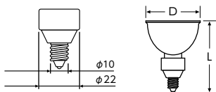
口金:EZ10 単位:mm 寸法図
