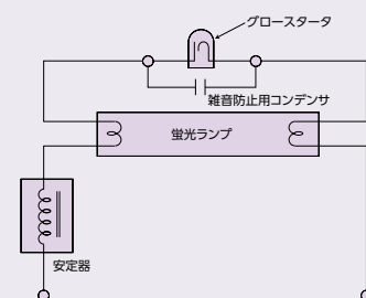
スタータ形蛍光灯の基本点灯回路
