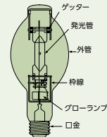
高圧ナトリウムランプの構造図
