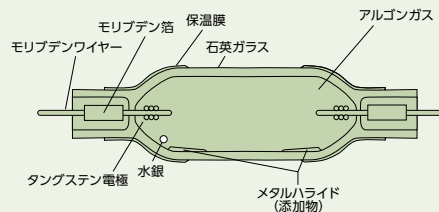
メタルハライドランプの発光管
