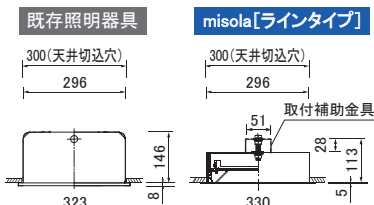
misola [ラインタイプ] 2台連結
