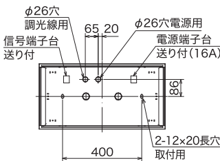
壁埋込施工時
