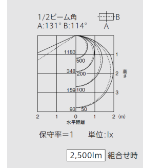
直付形下面開放タイプ2灯用 EL-LYX4062
