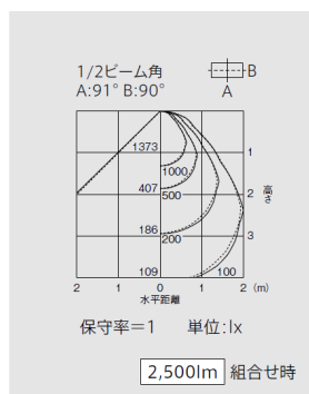
埋込形300幅ブラケットカバータイプ 2灯用 EL-LFB4552
