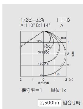
埋込形220幅ワゴン取付 可能タイプファインペ-ス2灯用 EL-LYB4002
