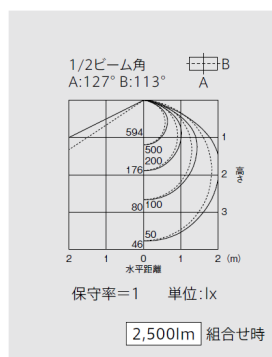
埋込形150幅ワゴン取付 可能タイプファインペ-ス1灯用 EL-LYB4001
