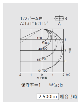
埋込形300幅ワゴン取付 可能タイプファインペ-ス2灯用 EL-LFB45122
