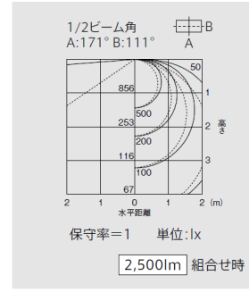
直付形逆富士タイプ2灯用 ﾌﾟﾙｽｲｯﾁ付 EL-LKV4342
