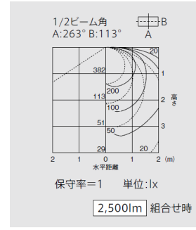
直付形片反射笠タイプ1灯用 EL-LFV4901
