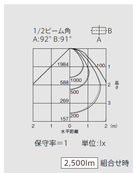
埋込形300幅ブラケットカバータイプ 3灯用 EL-LFB4553
