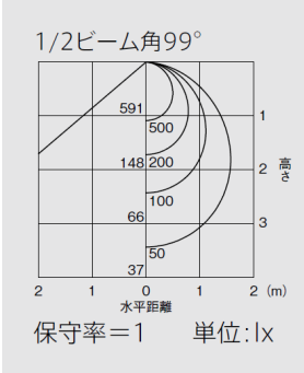
3000Kタイプ EL-V1510L/W
