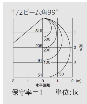
5000Kタイプ EL-V2010N/W
