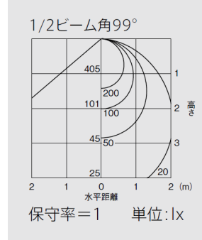
5000Kタイプ EL-V1010N/W
