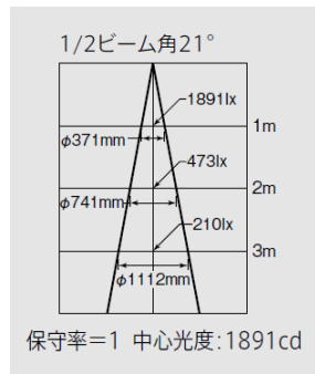
5000Kタイプ EL-V602W/W
