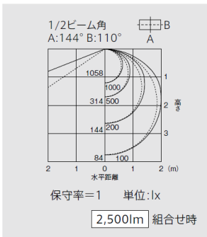
埋込形300幅2灯用 EL-LYWB41732
