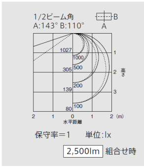
直付形反射笠タイプ2灯用 EL-LYWH4012A
