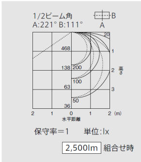
直付形片反射笠タイプ1灯用 EL-LYWF4021
