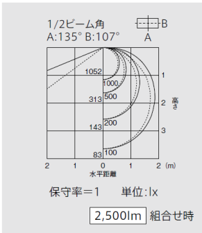
直付形反射笠タイプ2灯用 EL-LYEH4012A
