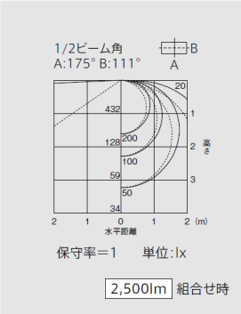
直付形逆富士タイプ1灯用 EL-LKV4371
