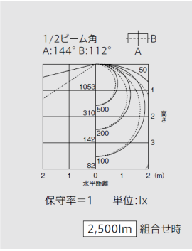
直付形反射笠タイプ2灯用 EL-LFH4932
