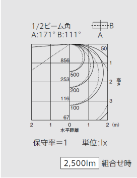
直付形逆富士タイプ2灯用 EL-LKV4392
