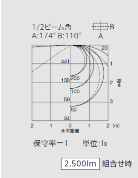
直付形トラフタイプ1灯用 EL-LKL4911
