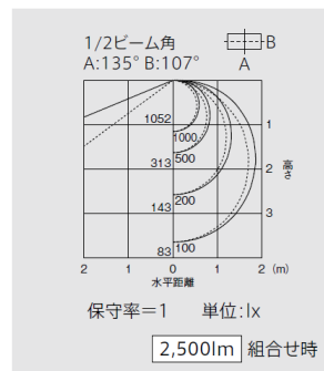
直付形反射笠タイプ2灯用 EL-LYEH4012A
