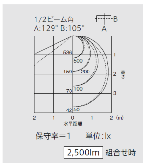
直付形反射笠タイプ1灯用 EL-LYEH4011A
