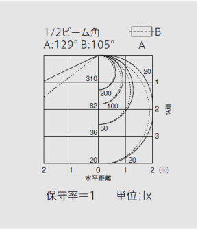
直付形反射笠タイプ1灯用 EL-LEH2041
