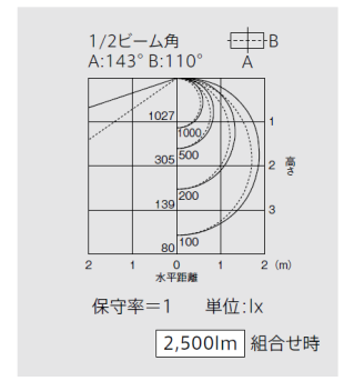
直付形反射笠タイプ2灯用 EL-LYWH4012A
