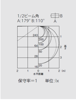
直付形逆富士タイプ 1灯用 フルスイッチ付簡易連結具付 (1灯→消灯) EL-LKV2261
