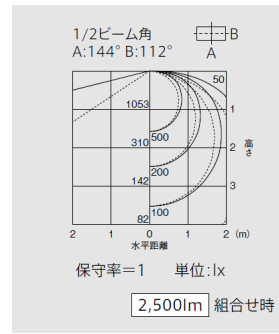
直付形反射笠タイプ2灯用 EL-LFH4902
