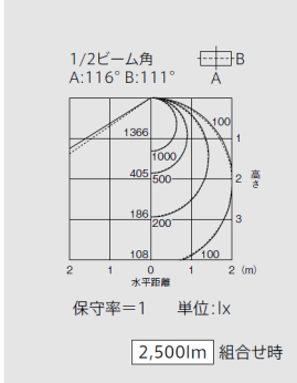
埋込形300ヘン皿カバータイプ 3灯用 EL-LFY4563
