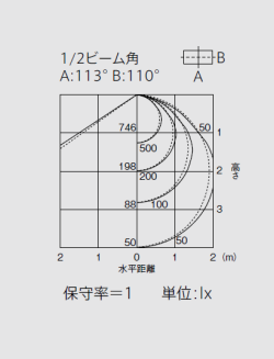
埋込形220幅ワゴン取付可能 タイプファインベース2灯用 EL-LYB2062
