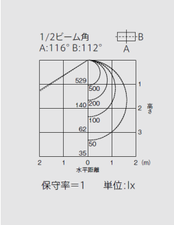
埋込形300幅ベージュ乳白カバータイプ 2灯用 EL-LFY2542
