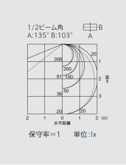
直付形逆富士タイプ 1灯用 簡易連結具付 EL-LKV2251
