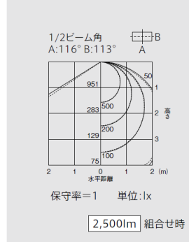
埋込形300幅ヘン皿カバータイプ 2灯用 EL-LFY4562
