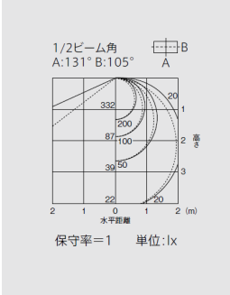
直付形反射笠タイプ 1灯用 EL-LFH2571
