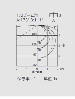
直付形逆富士タイプ 2灯用 フルスイッチ付簡易連結具付 (2灯→消灯) EL-LKV2262
