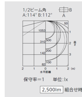
直付形反射笠タイプ2灯用 ﾌﾟﾙｽｲｯﾁ付 EL-LFH4912
