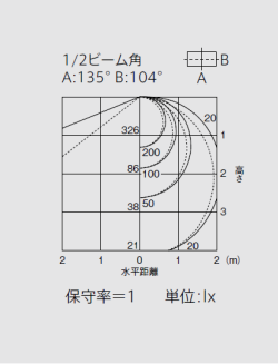
直付形トラタイプ 1灯用 EL-LKL2571
