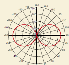
LHT58L-G-E39/1000 (電球色)
