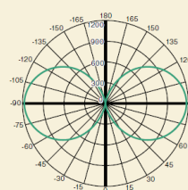
LHT58N-G-E39/1000 (昼白色)
