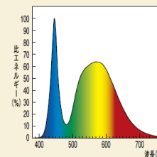
LHT58N-G-E39/1000 (昼白色)
