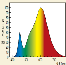
LHT58L-G-E39/1000 (電球色)
