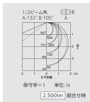
直付形 トラフタイプ1灯用 EL-LYEL4011A
