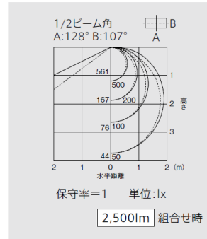
直付形 反射笠タイプ1灯用 EL-LYWH4011A
