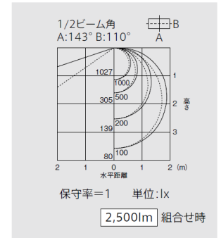
直付形 反射笠タイプ2灯用 EL-LYWH4012A
