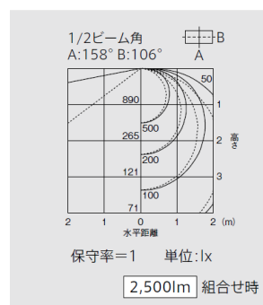
直付形 逆富士タイプ2灯用 EL-LYEV4012A
