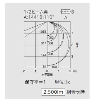
埋込形 300幅2灯用 EL-LYWB41732
