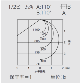
3000K 100%時
