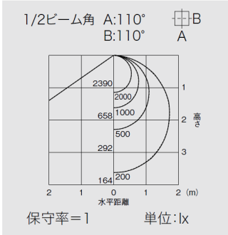
全灯(混光)時
