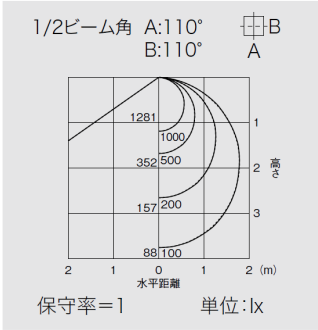
5000K 100%時
