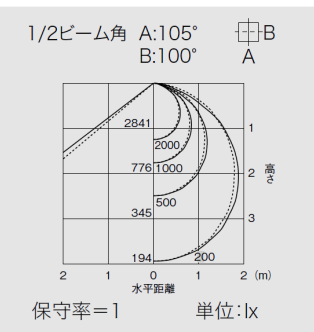
全灯(混光)時
