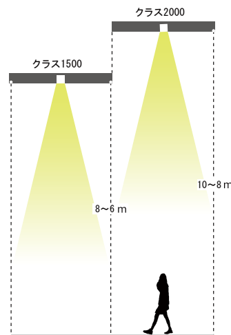
■ 出カクラスと天井高の目安
