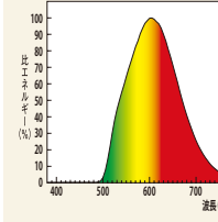
低誘虫用 LDL40T・Y/17/20・G3
