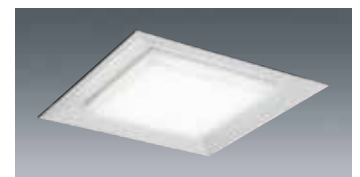
リニューアル対応タイプ (埋込形 □600)
