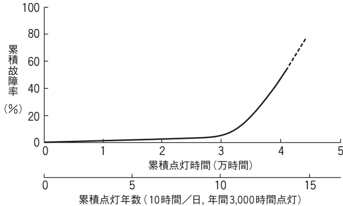
図 1 照明器具の累積故障率
