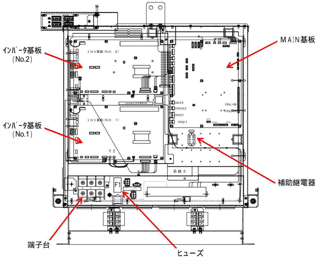
制御箱 系統2 内部配置図 (手前側)
