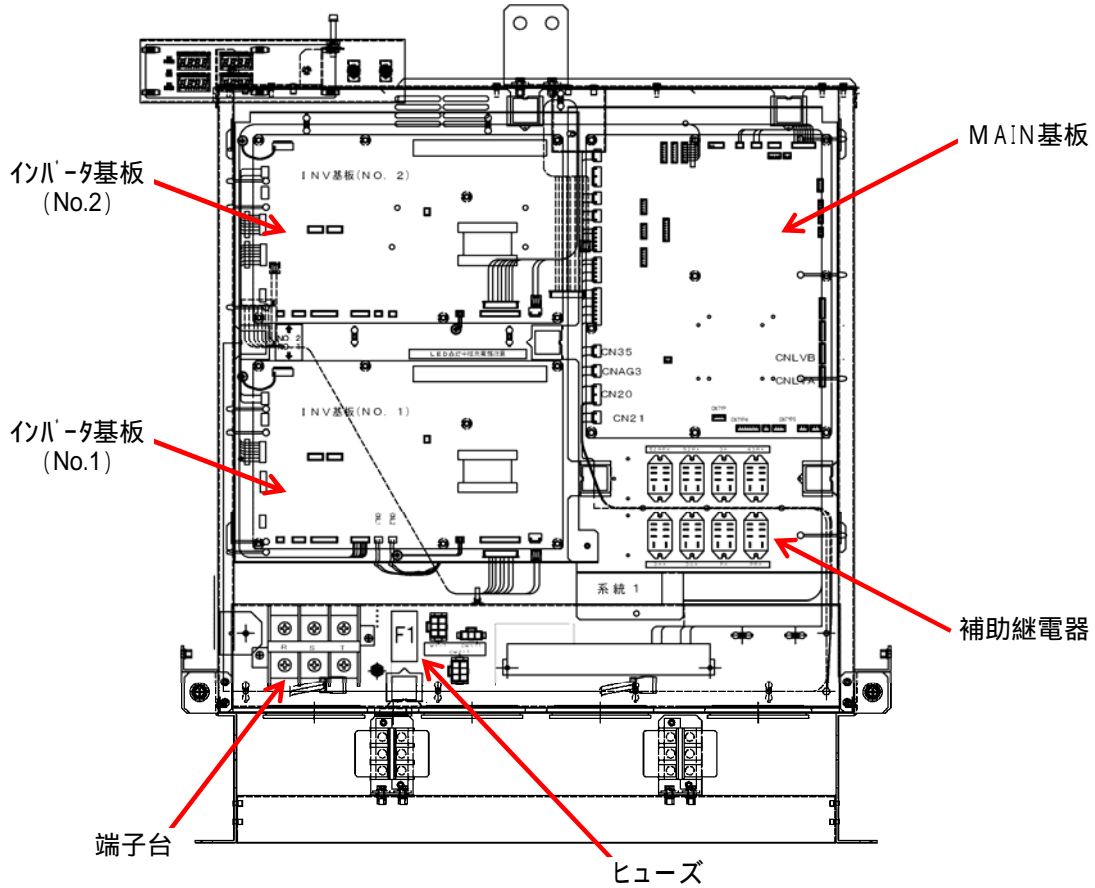
制御箱 系統1 内部配置図 (手前側)
