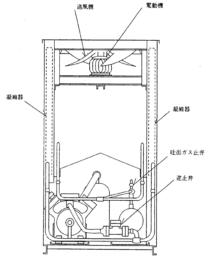
側面図
