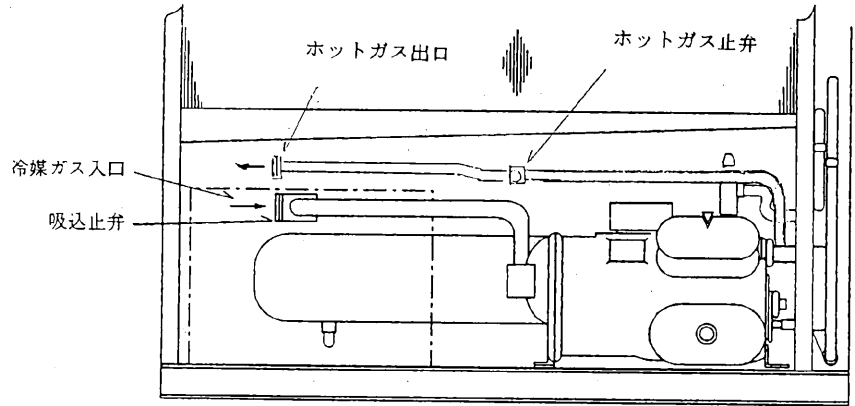
正面図
