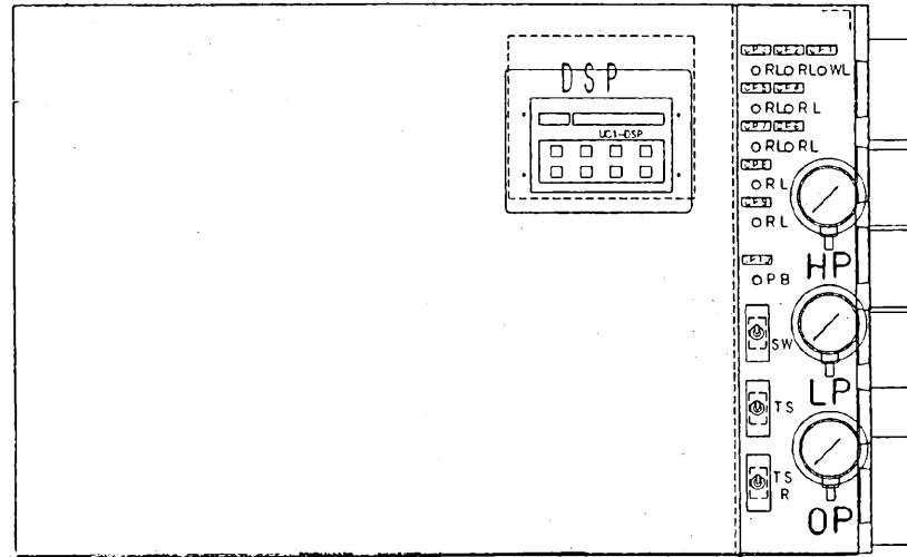
制御箱正面
