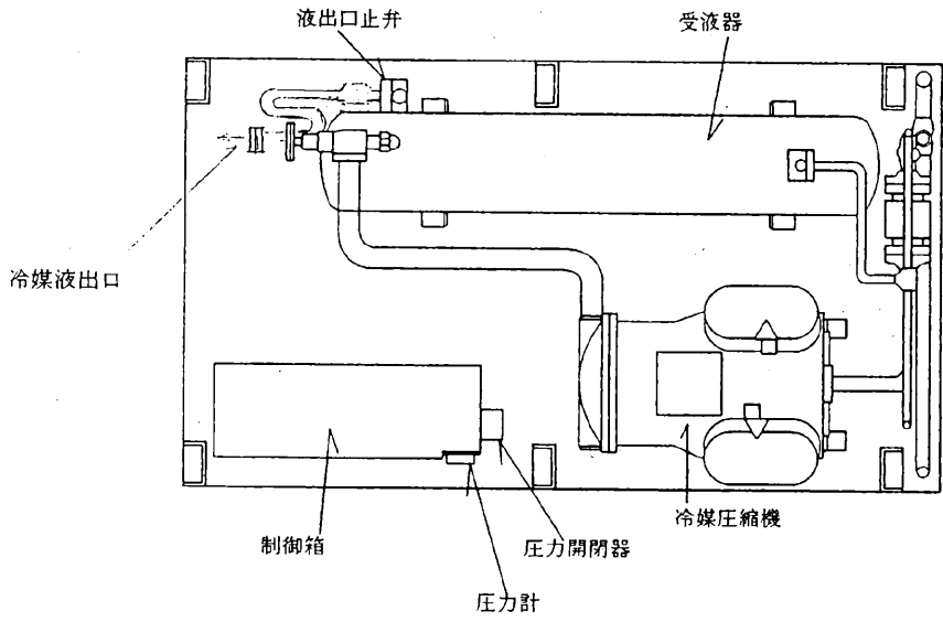
平面図 (機械室)
