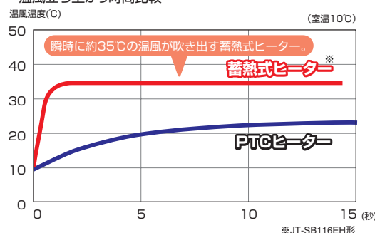
■蓄熱式『即暖ヒーター』とPTCヒーターの温風立ち上がり時間比較
