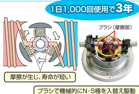
■整流子モーター
