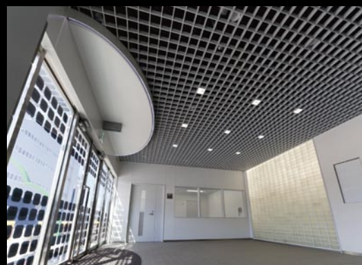
エントランスホール ルーバ天井内に特注ダウンライトを設置し、建築空間と一体化した照明計画を行っています。
