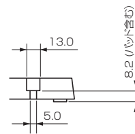
転倒防止固定ネジ穴部 断面図
