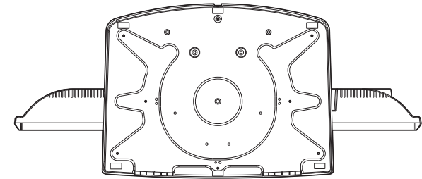
底面
