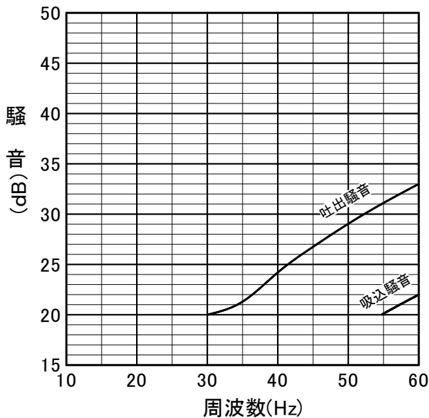
■ 騒音特性図
