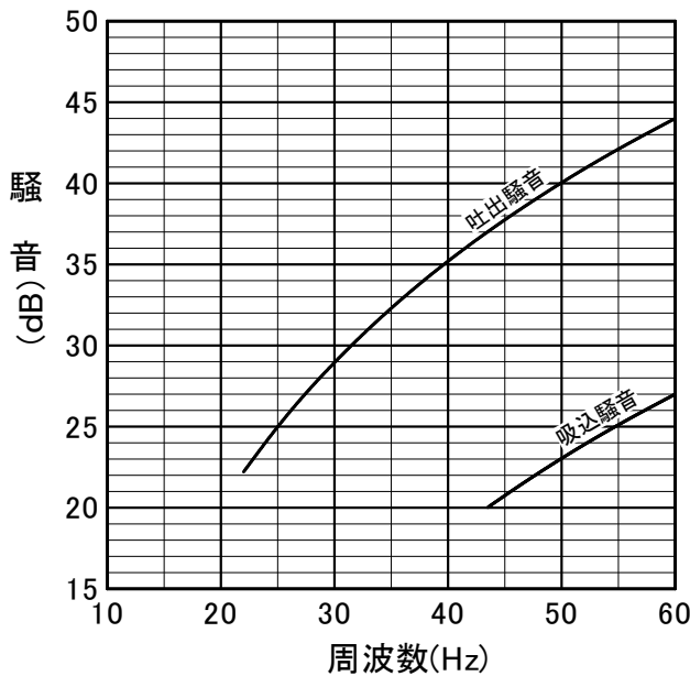
■ 騒音特性図
