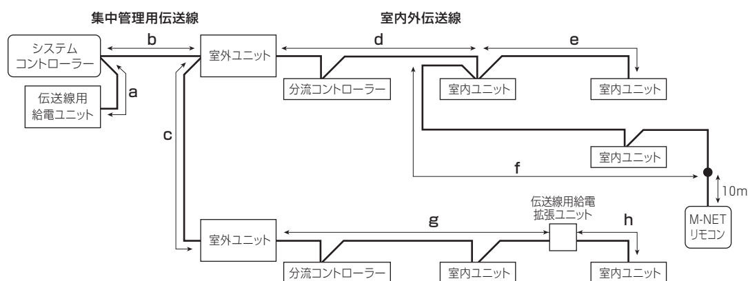
【図 2-1】 M-NET伝送線の配線図例
