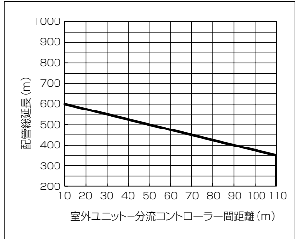
【PURY-P560, 630SCM-G】
