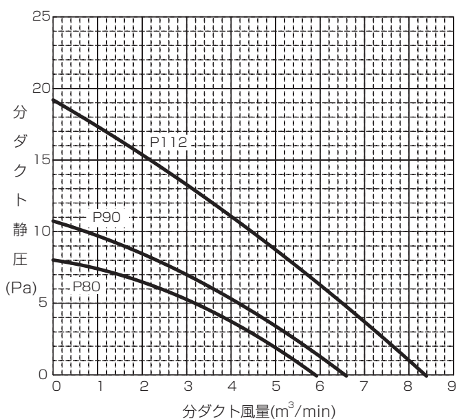
■PLFY-P80・P90・P112LM-G
