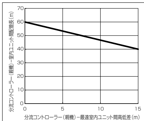
図1. 分流コントローラー-室内ユニット高低差と枝管長
