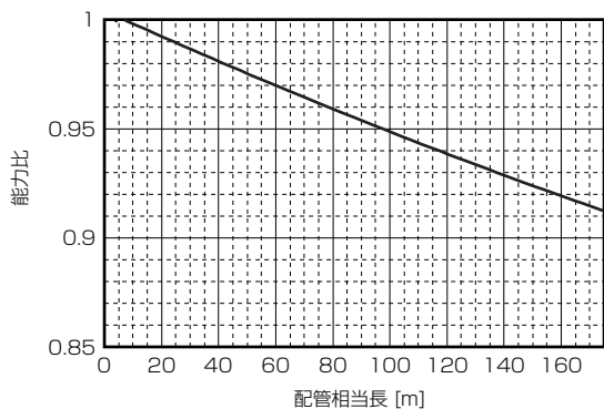
■PURY-P224CM-G (-BS, -BSG)
