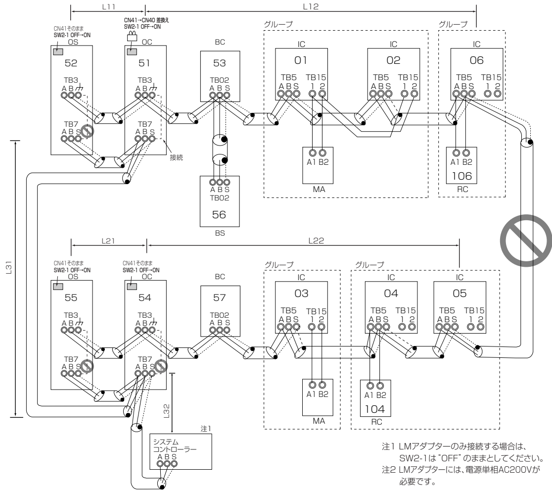
制御線配線例
