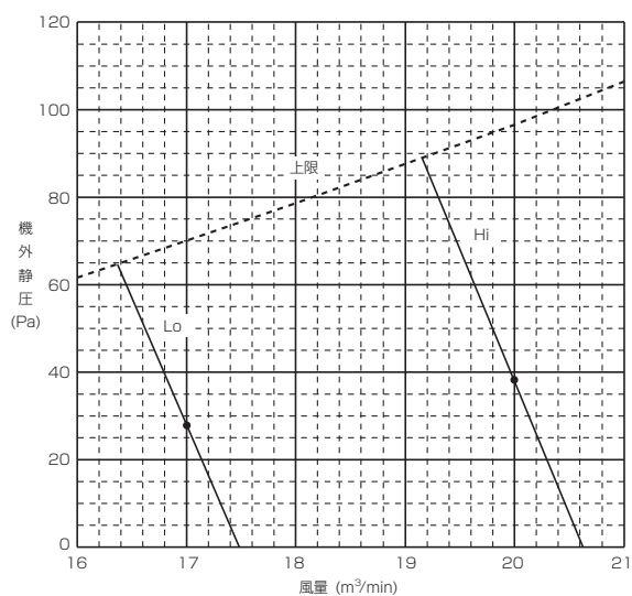
■PLFY-P45・56CLM-G
