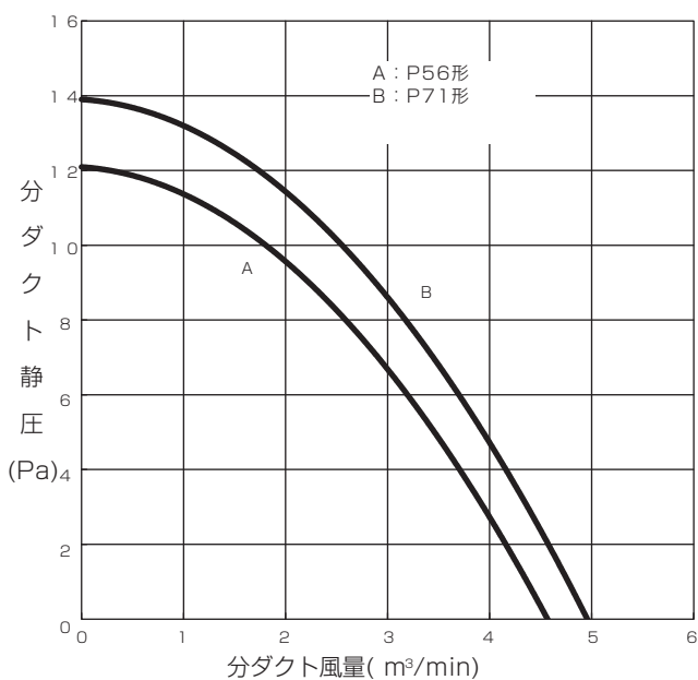
■PLFY-P56・P71LM-G
