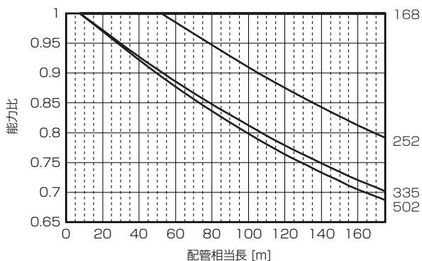
■PURY-P335CM-G (-BS, -BSG)
