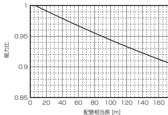
■PURY-P280, 335CM-G (-BS, -BSG)
