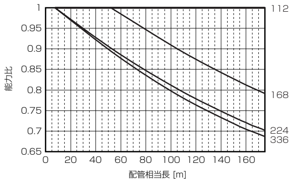
■PURY-P224CM-G (-BS, -BSG)
