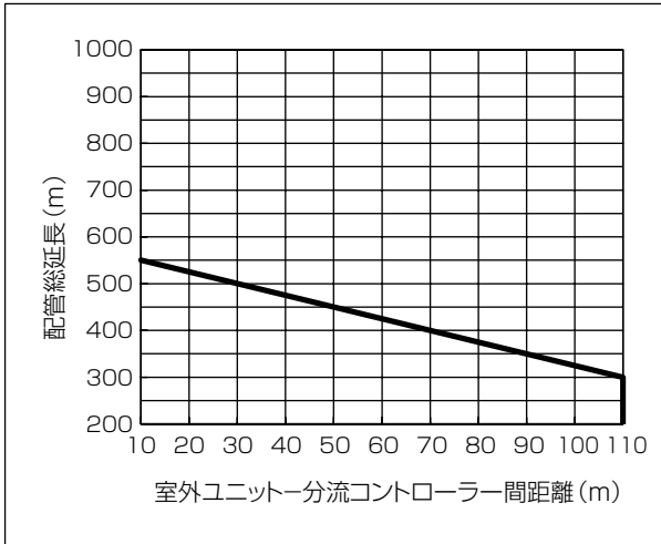
【PURY-P500SCM-G】
