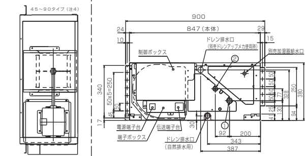
サービススペース詳細図
