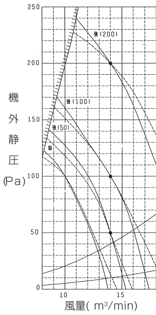
■PEFY-P45・56M-G
