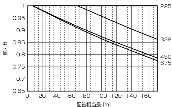
■PURY-P450CM-G (-BS, -BSG)
