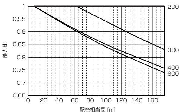
■PURY-P400CM-G (-BS, -BSG)
