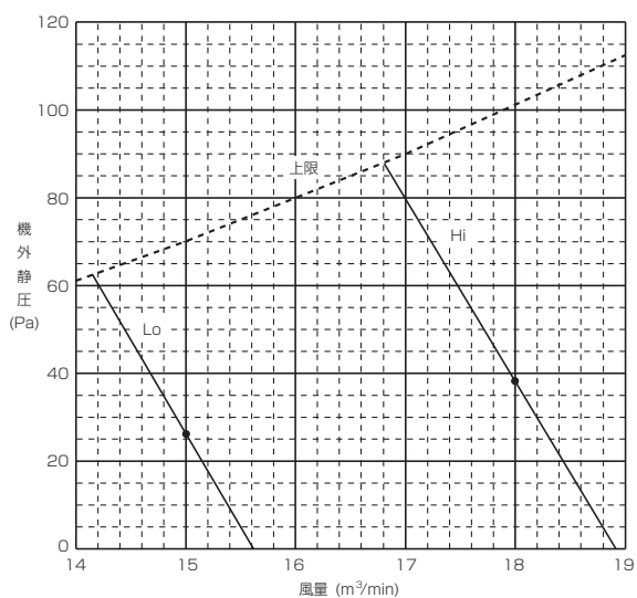
■PLFY-P36CLM-G
