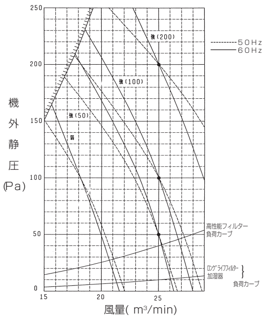
■PEFY-P90M-G
