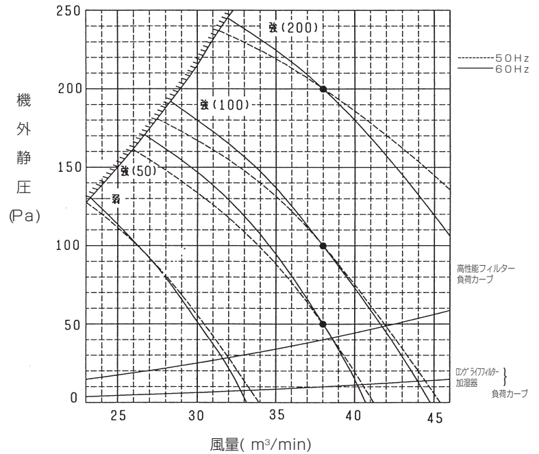
■PEFY-P112・140M-G
