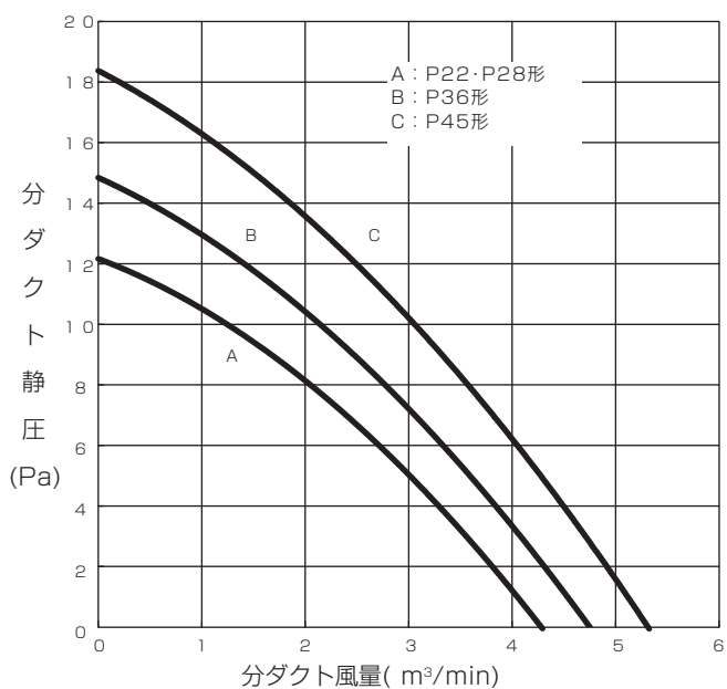
■PLFY-P22・P28・P36・P45LM-G
