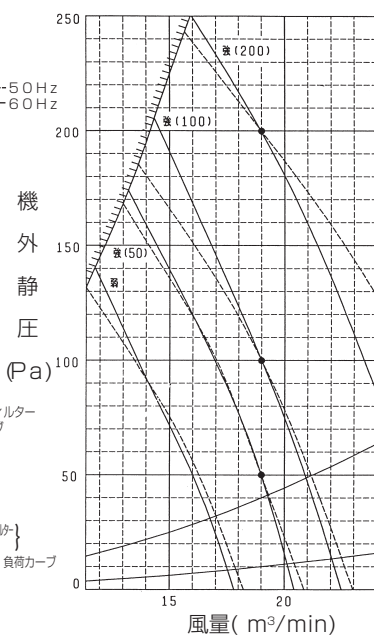
■PEFY-P71M-G
