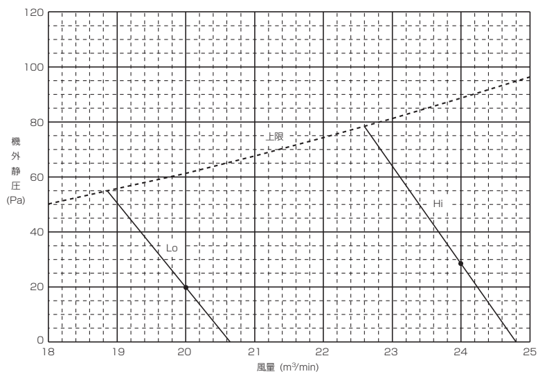
■PLFY-P71・80CLM-G
