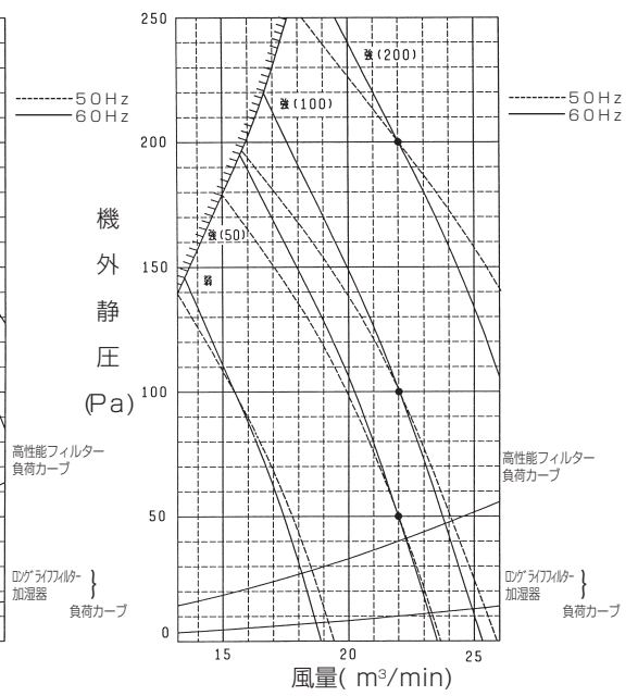
■PEFY-P80M-G
