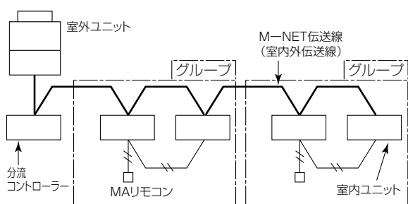
<MAリモコンを使用した場合>
