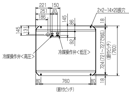
下面から見た図
