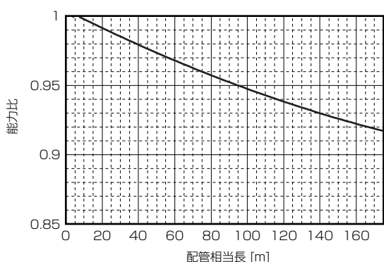
■PURY-P400CM-G (-BS, -BSG)
