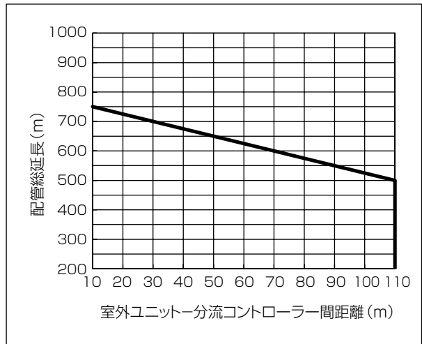
【PURY-P800, 850, 900SCM-G】
