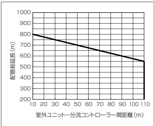
【PURY-P690, 730SCM-G】
