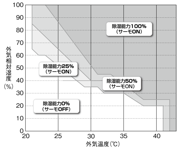
■除湿能力マップ(目標湿度到達時)
