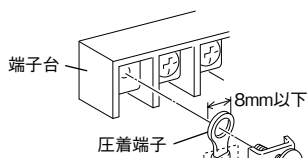
圧着端子 接続例
