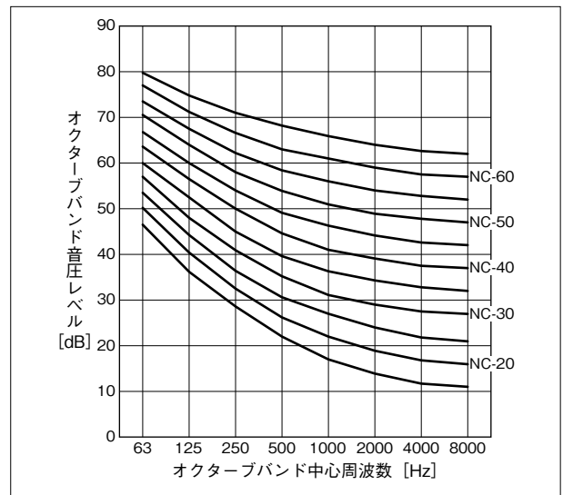
■ N-C曲線
