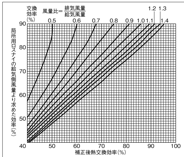
■局所用ロスナイ効率補正曲線 (温度交換効率)
