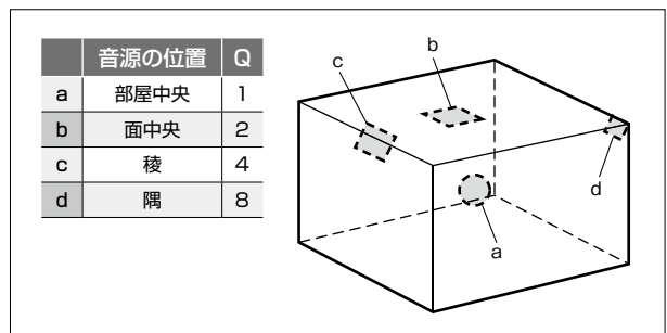
■ 図-3 (音源の位置と指向係数Q)
