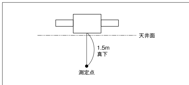
■図-2 天井埋込(天井埋込ダクト)形の場合
