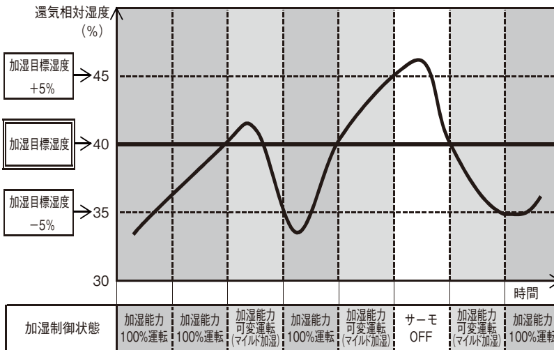
■ 加湿制御状態の切り換えイメージ
