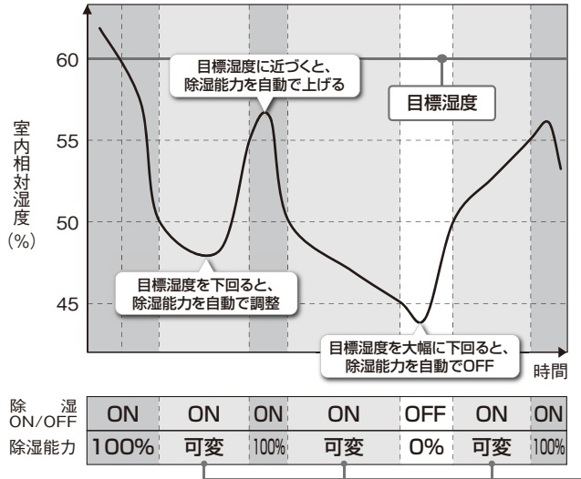
■「スマート除湿モード」運転イメージ (除湿目標湿度0.0125kg/kg(DA) (26℃、60%相当)の場合)
