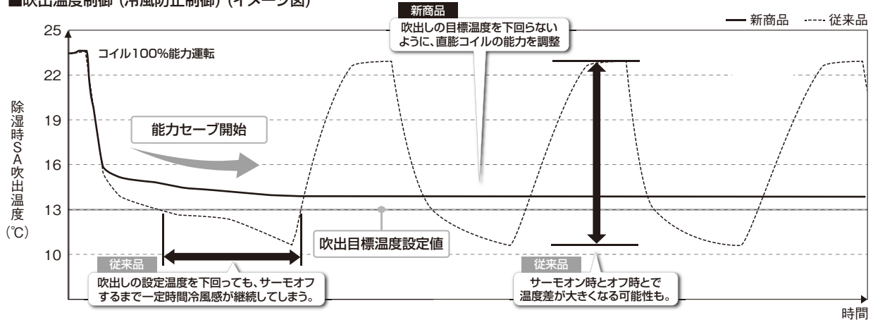
■吹出温度制御 (冷風防止制御) (イメージ図)
