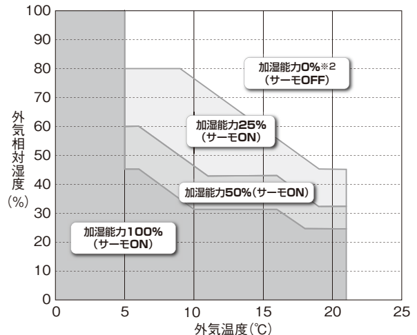
■加湿能力マップ(目標湿度到達時)
