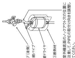
PAC-SG81, 82DRの場合
