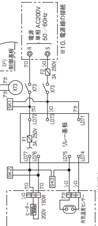
※11. ベースヒーター、外気温度センサーの接続
