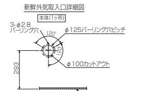
新鮮外気取入口詳細図
