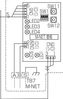
M-NET アダプター接続時
