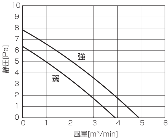
PS-RP56GA5
