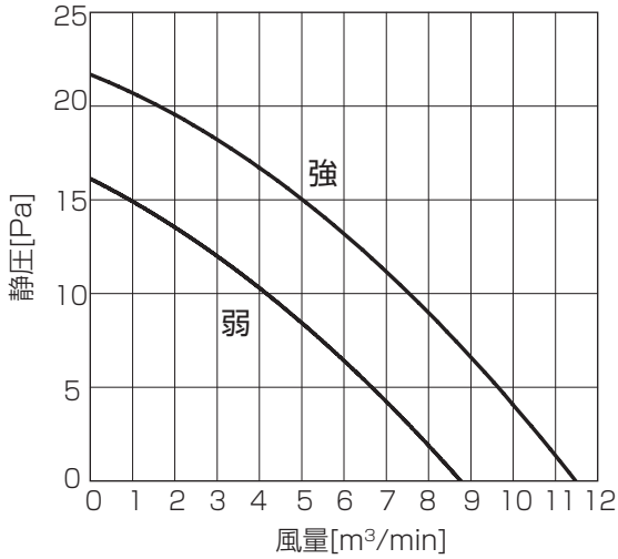
PS-RP160KA6
