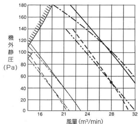
< 角形ダクト仕様 > PD-RP112FA6
