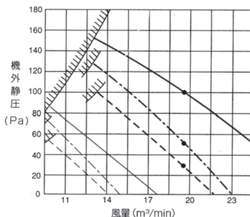
< 角形ダクト仕様 > PD-RP80FA6
