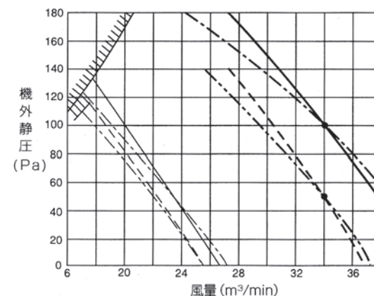
< 角形ダクト仕様 > PD-RP140FA6, PD-RP160FA6
