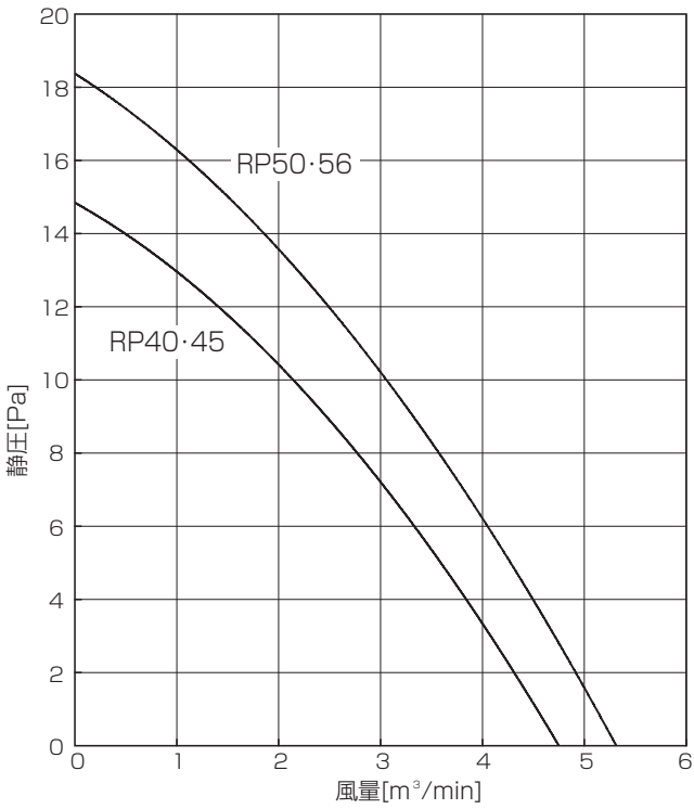
PL-RP40LA6, PL-RP56LA6
