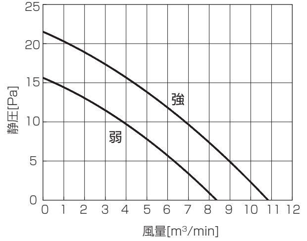
PS-RP140KA6
