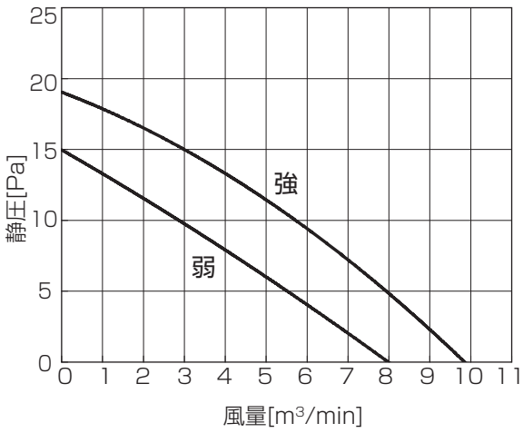
PS-RP112KA6
