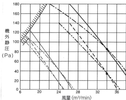
< 円形ダクト仕様 > PD-RP140FA6, PD-RP160FA6
