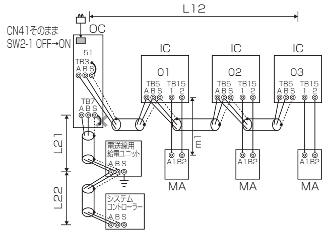
上位系を接続する場合(室内外アドレス手動設定)
