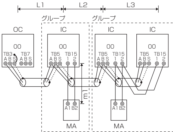
室内外自動アドレス立ち上げ
