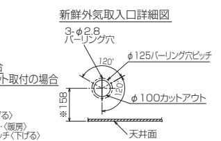
新鮮気取入口詳細図
