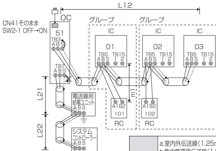
M-NETリモコンを接続する場合(室内外アドレス手動設定)
