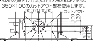
分ダクト接続口詳細図(両側面)
