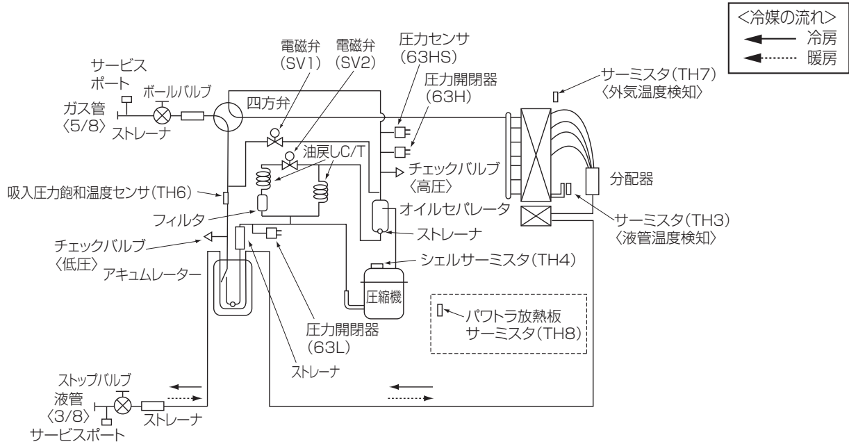
● 冷媒配管サイズ < フレア接続サイズ >
