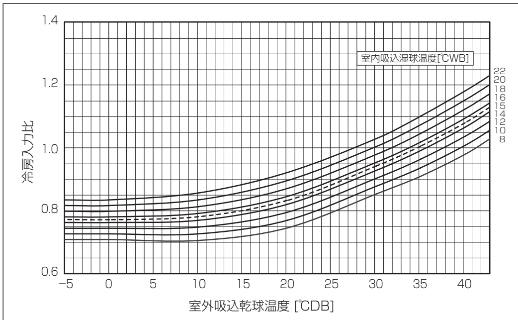
■冷房入力線図 PU(Z)G-P・MHA12
