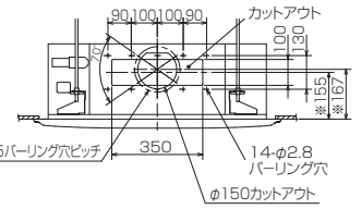
分ダクト接続口 分ダクト接続口詳細図(両側面)
