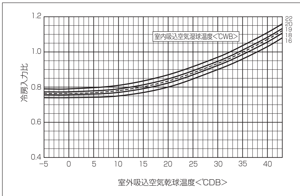
■冷房入力線図 PUZ-SRP・HA12
