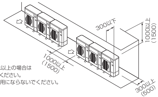
(5) 1台多列設置の場合
