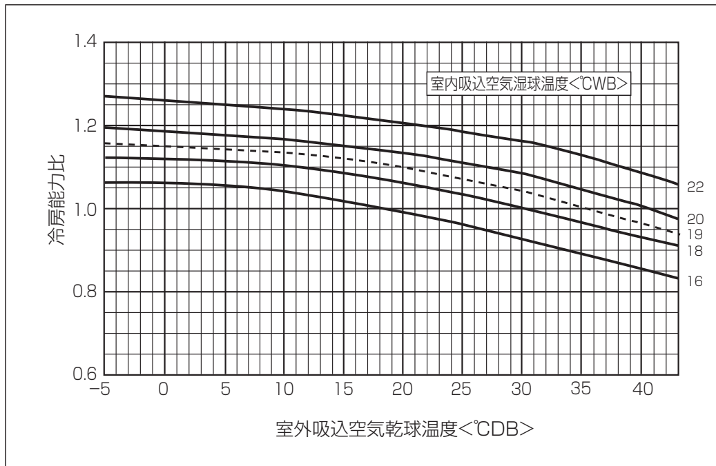
■冷房能力線図 PUZ-SRP・HA12
