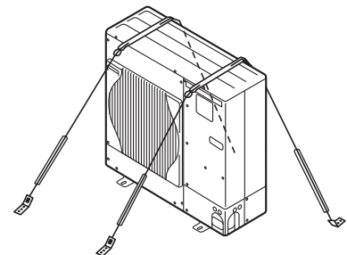
室外ユニットをワイヤーと金具で追加固定します。
