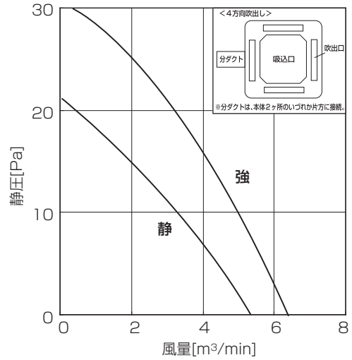
●4方向吹出し(ベーン水平)角形ダクト 1方向分岐
