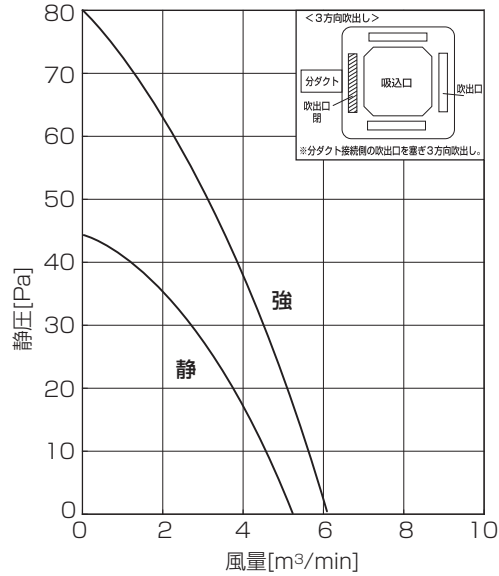
●3方向吹出し(ベーン水平)丸形ダクト 1方向分岐
