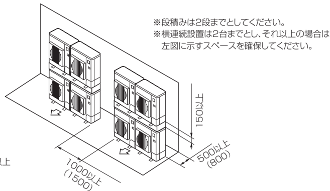
(7) 段積み設置の場合
