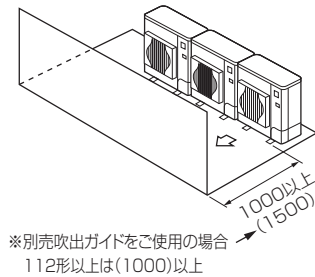
(3) 正面に障害物がある場合 (背面、側面、上方は開放)
