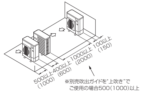
(5) 1台多列設置の場合
