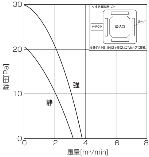
●4方向吹出し(ベーン水平)丸形ダクト 1方向分岐
