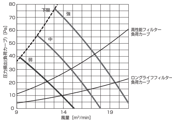
PD-RP40,56GA9 (機外静圧 30Pa)
