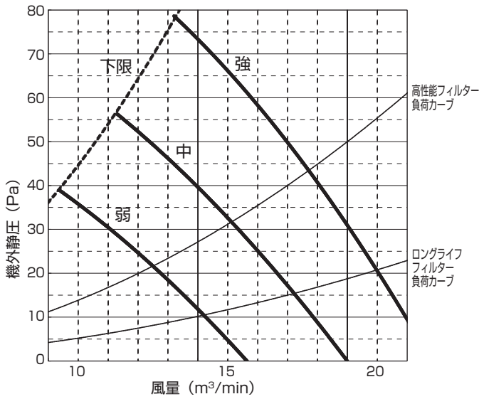
PE-RP56DA9 (機外静圧 50Pa)
