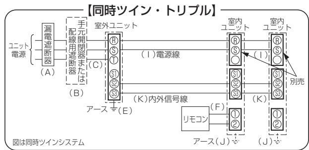
図は同時ツインシステム
