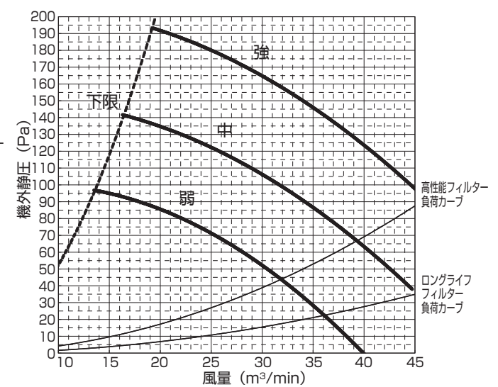
PE-RP160DA9(機外静压 150Pa)
