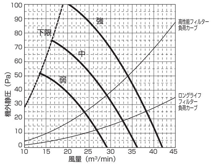
PE-RP112DA9 (機外静压 50Pa)
