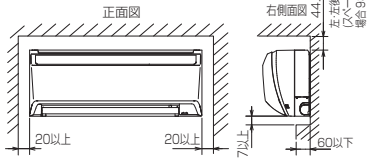
据付所要スペース(室内ユニット)
