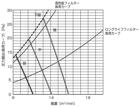
PD-RP40,56GA9 (機外静圧 70Pa)
