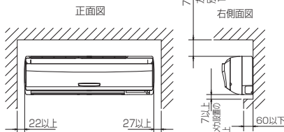
据付所要スペース(室内ユニット)
