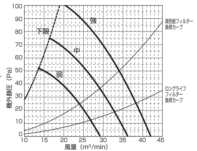
PE-RP160DA9(機外静压 50Pa)
