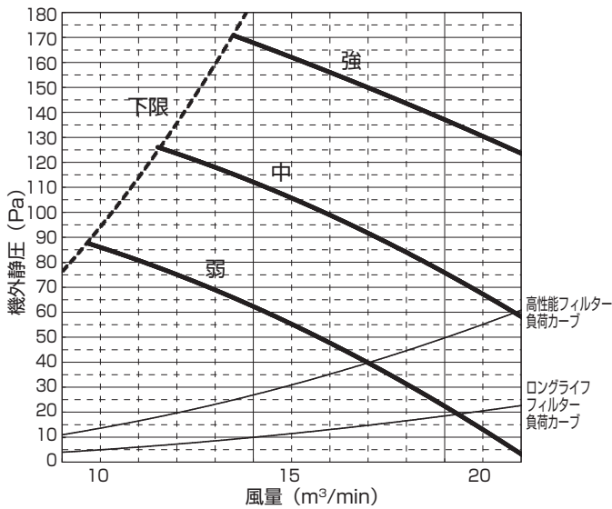
PE-RP56DA9 (機外静圧 150Pa)
