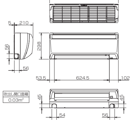
室内ユニット外形図
