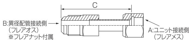
<リブレース異径ジョイント外形図>
