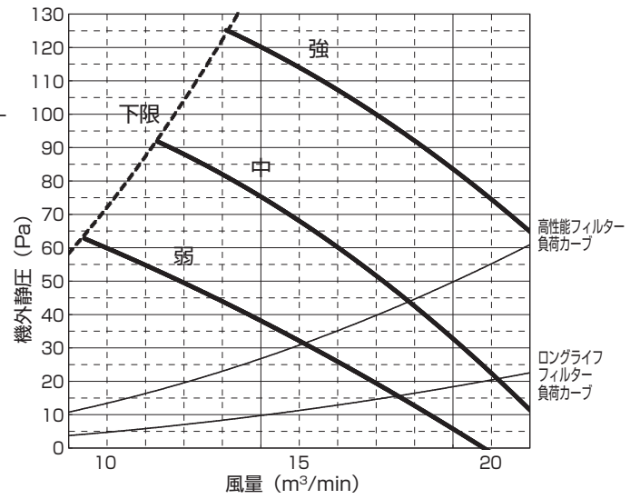
PE-RP56DA9 (機外静圧 100Pa)
