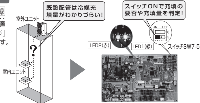
室外制御基板 *この写真はP80~P160形用です。
