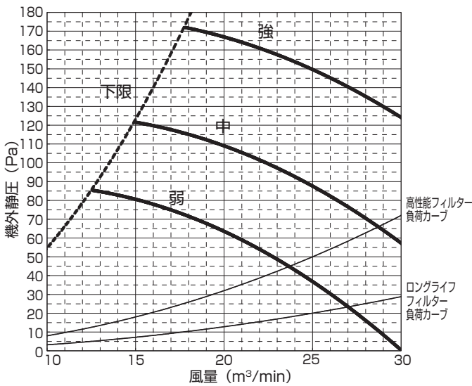
PE-RP80DA9 (機外静压 150Pa)
