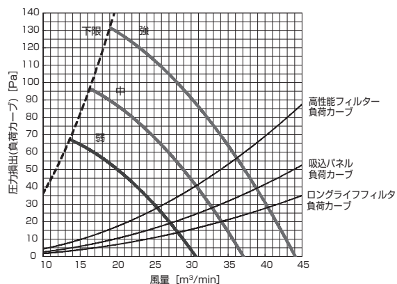
PD-RP160GA9 (機外静圧 70Pa)
