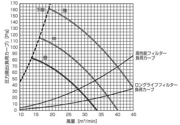
PD-RP140GA9 (機外静圧 50Pa)
