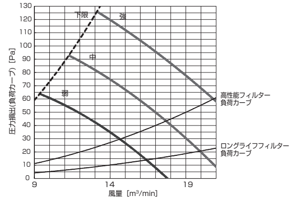
PD-RP40,56GA9 (機外静圧 50Pa)
