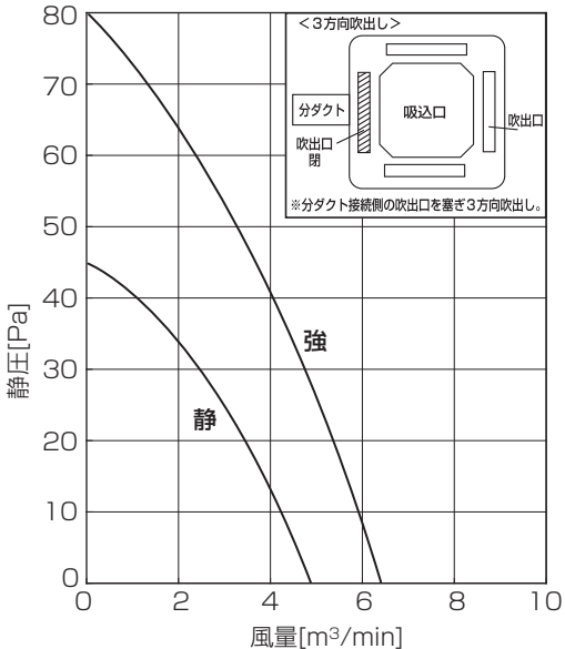
●3方向吹出し(ペーン水平)丸形ダクト 1方向分岐
