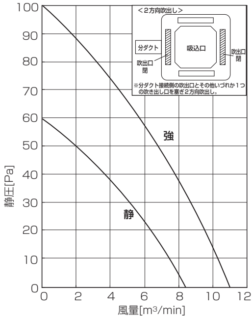
●2方向吹出し(ペーン水平)角形ダクト 1方向分岐
