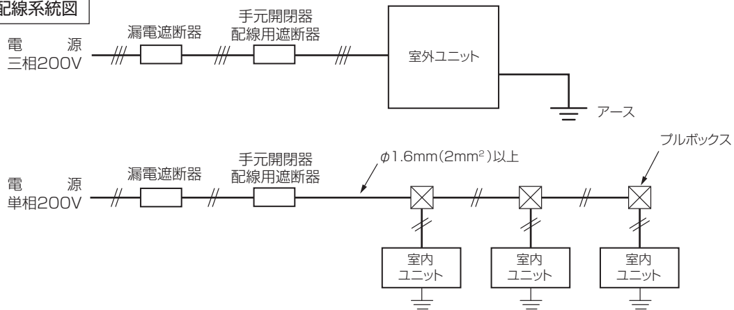
主電源の配線系統図
