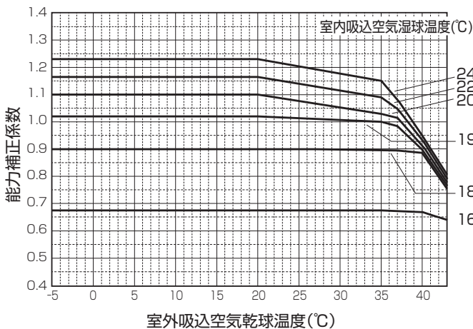
<図1> 冷房能力・入力補正
