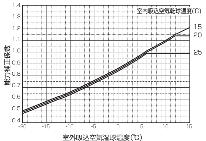
<図2> 暖房能力・入力補正
