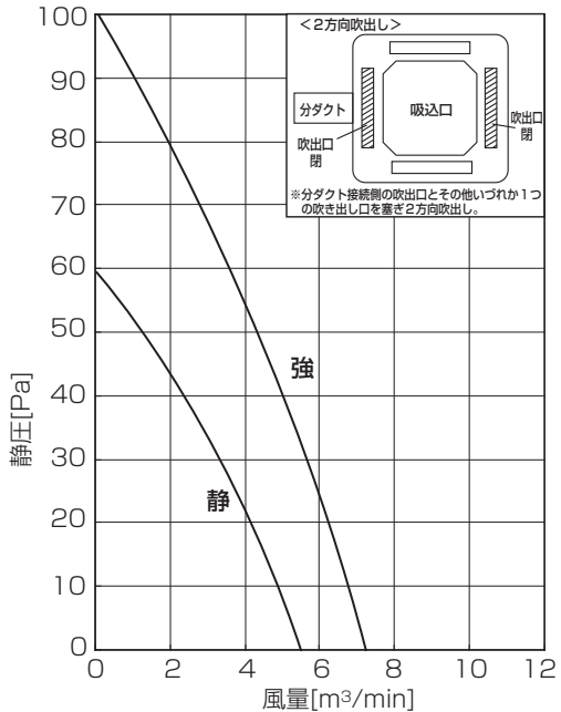
●2方向吹出し(ペーン水平)丸形ダクト 1方向分岐
