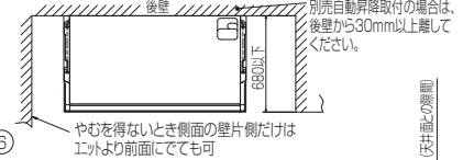
室内ユニット周囲必要空間
