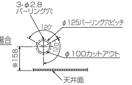
新鮮気取入口詳細図
