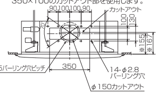
新鮮気取入口詳細図
