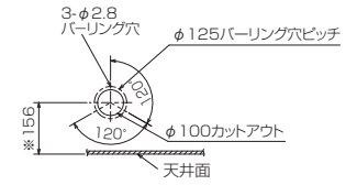
分ダクト接続口詳細図(両側面)
