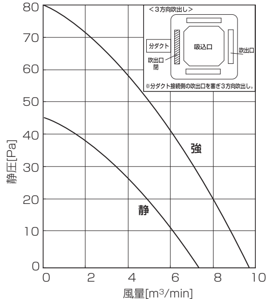
●3方向吹出し(ペーン水平)角形ダクト 1方向分岐
