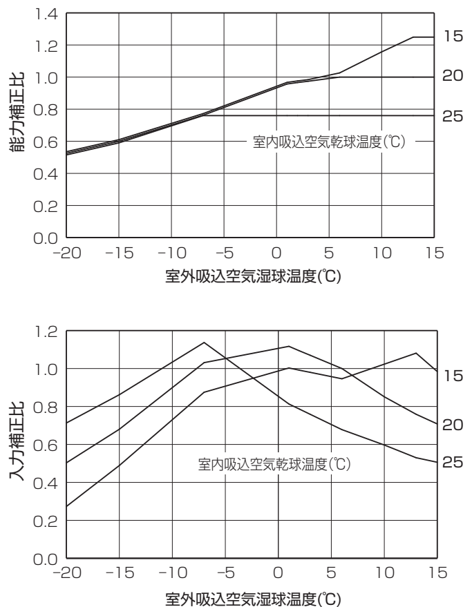
< 図 2 > 暖房能力・入力補正
