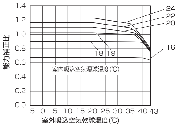
< 図 1 > 冷房能力・入力補正
