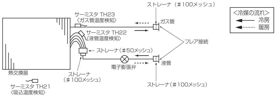
●冷媒配管サイズ<フレア接続サイズ>
