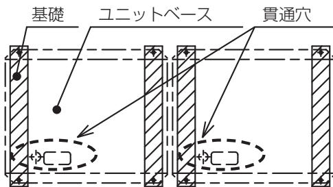
基礎をユニット奥行き方向に施工する場合
