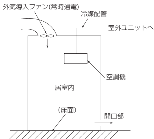
図1 常時換気システム（外気導入の例）
