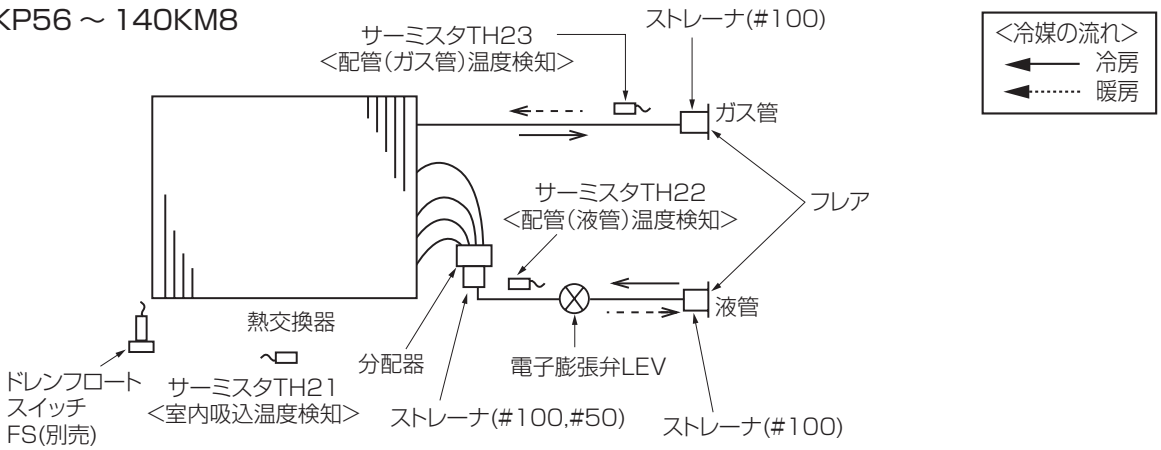
●冷媒配管サイズ<フレア接続サイズ>
