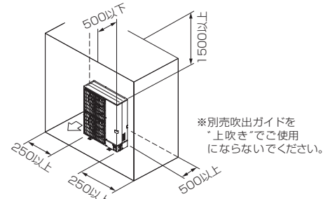
(6) 背面と側面および上方に障害物がある場合 (正面は開放)
