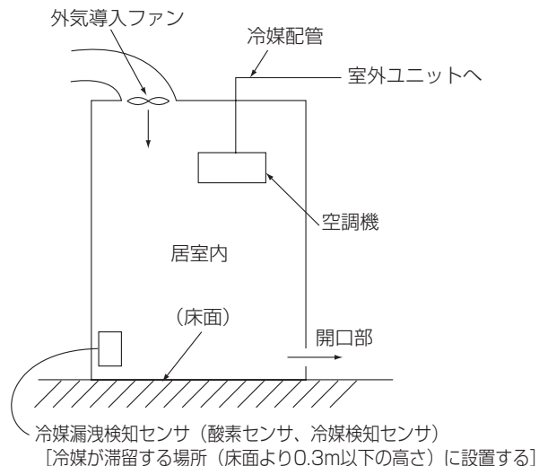
図2 センサ連動システム（外気導入の例）
