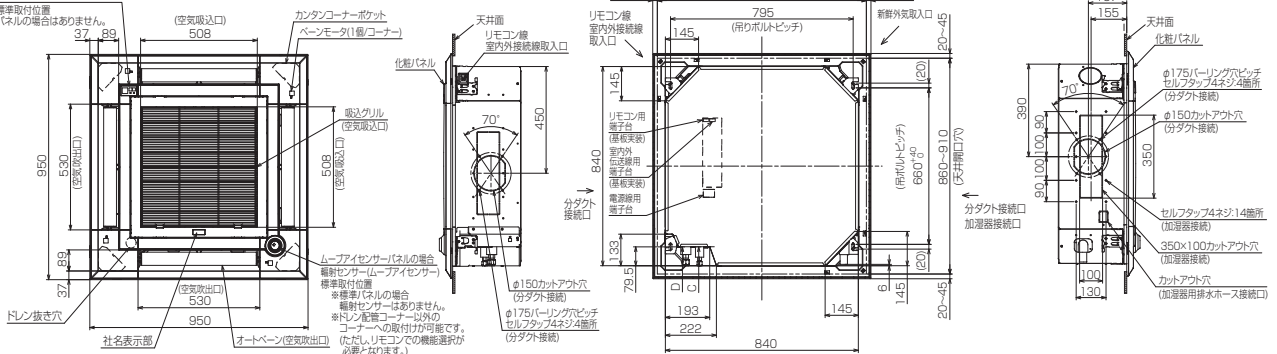
●機種ごとの能力は下記による PLZ-KP-EM: 56/71/80/90/112/140
