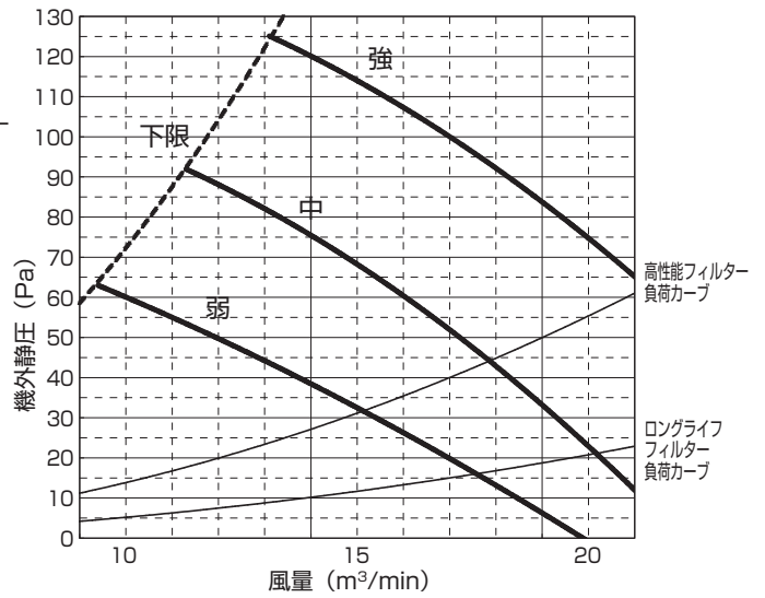
PE-RP50DA 10(機外静圧 100Pa)
