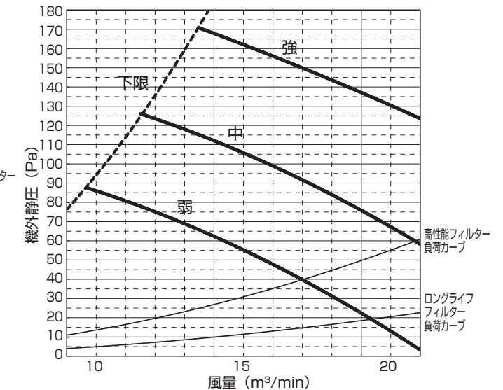
PE-RP56DA 10(機外静圧 150Pa)
