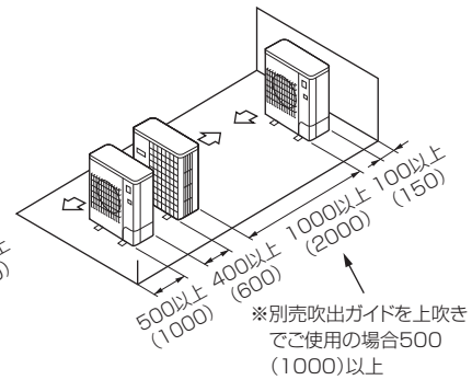
(5) 1台多列設置の場合
