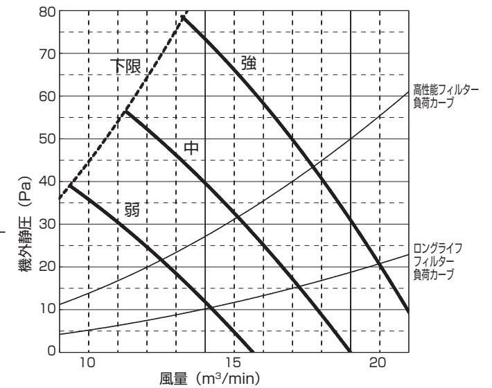
PE-RP56DA 10(機外静圧 50Pa)
