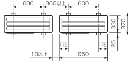
ZRMP112~160形の場合 ZRP/ERP224・280形の場合
