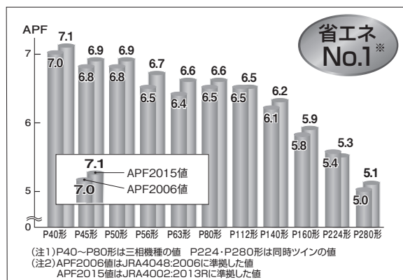
■能力別 APF 値(4 方向天井カセット形 50Hz)
