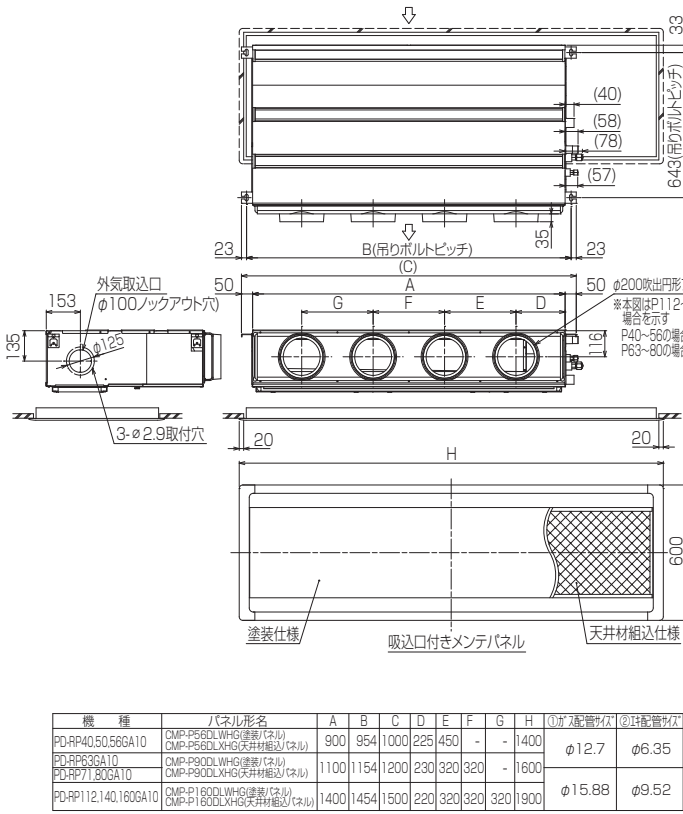
＜標準仕様(下吸込)＞
