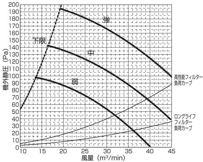
PE-RP140DA10(機外静压 150Pa)
