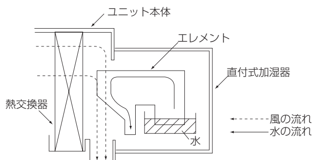
自然蒸発式の加湿メカニズム(直付式加湿器の場合)
