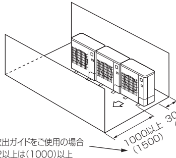
(4) 背面と正面に障害物がある場合 (側面、上方は開放)
