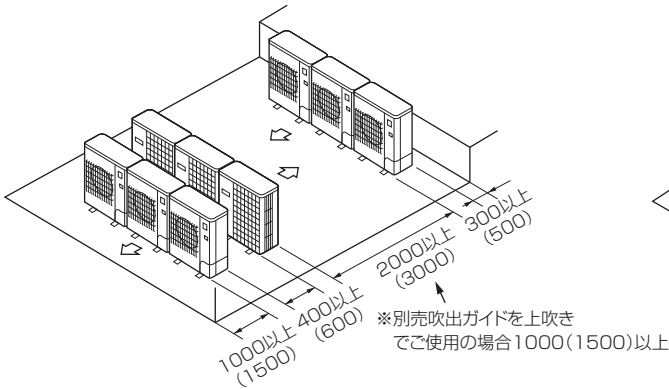
(6) 複数台多列設置の場合
