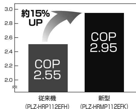
低外気温時(2℃)の省エネ性 ※2 (4方向天井カセット形)
