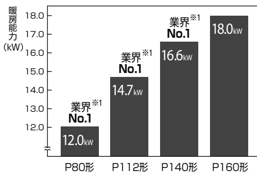
低外気温時(2℃)の暖房能力 ※2 (4方向天井カセット形)
