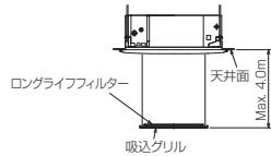
カタン自動パネル 吸込グリル昇降寸法
